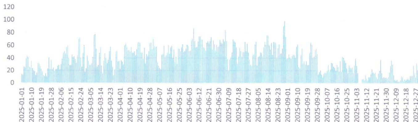
Слика 8. Приказ средњих дневних концентрација озона у 2025. години на мерном месту „Цара Душана“
