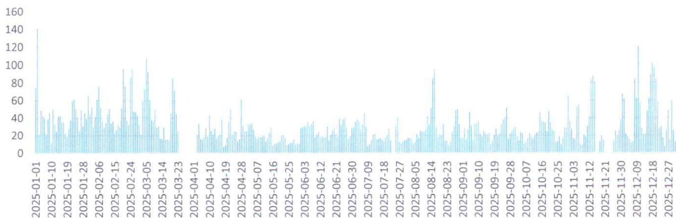
PM_{10} ( \mu g/m^3 ) за 24ч "Ватрогасни дом"
