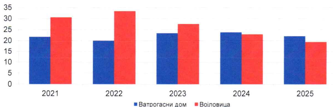
Средње годишње вредности PM_{2,5} ( \mu g/m^3 )
