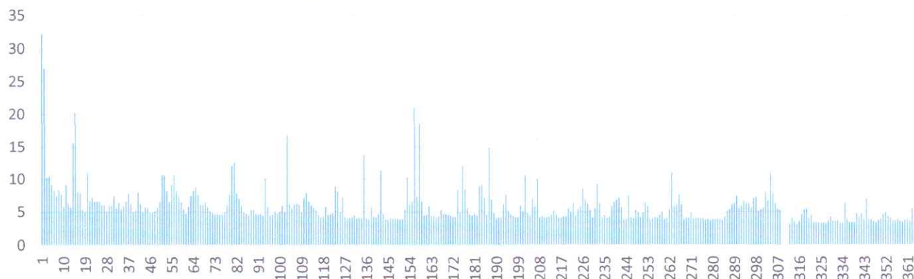
SO 2 (µg/m 3 ) за 24ч "Цара Душана"
