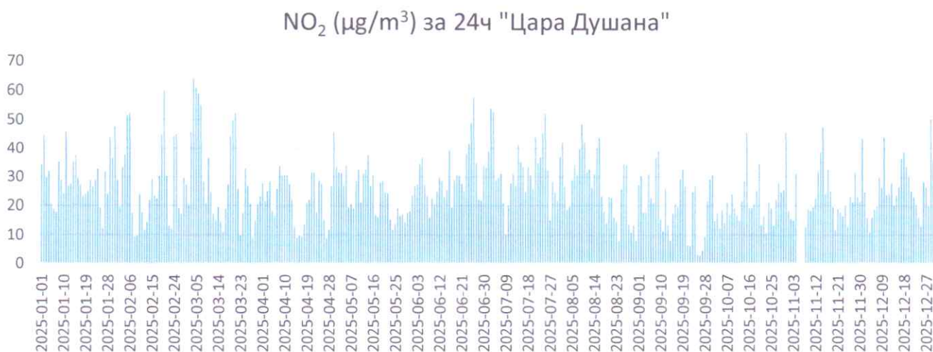
Слика 4. Приказ средњих дневних концентрација азотдиоксида у 2025. години на мерном месту „Цара Душана“
