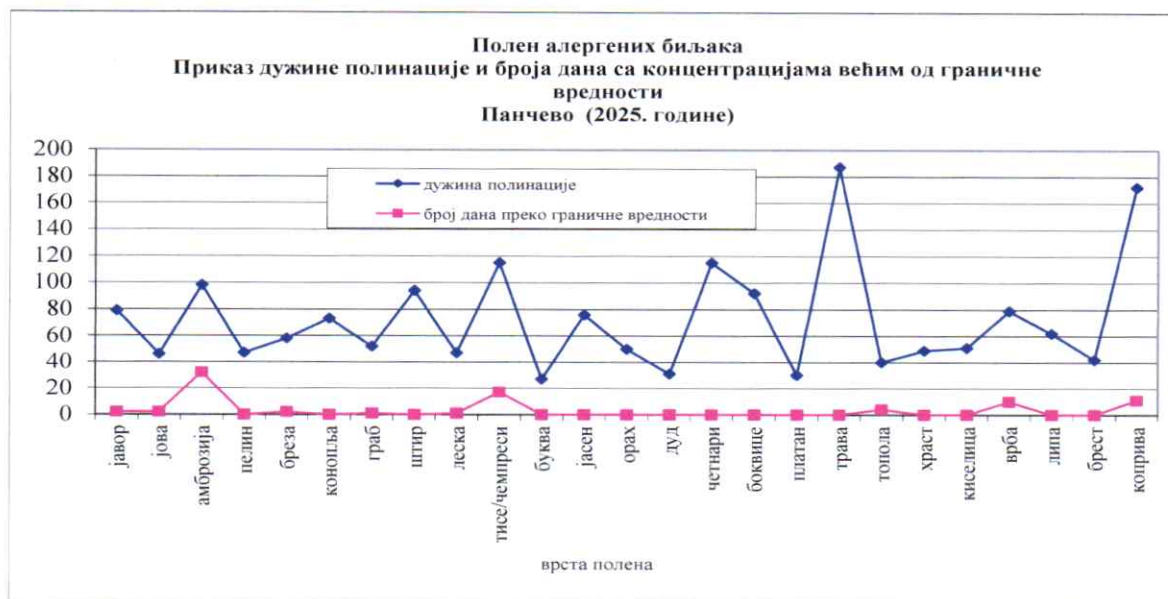
Слика 31. Дистрибуције дужине полинације и броја дана са концентрацијама изнад граничне вредности полена алергених биљака
