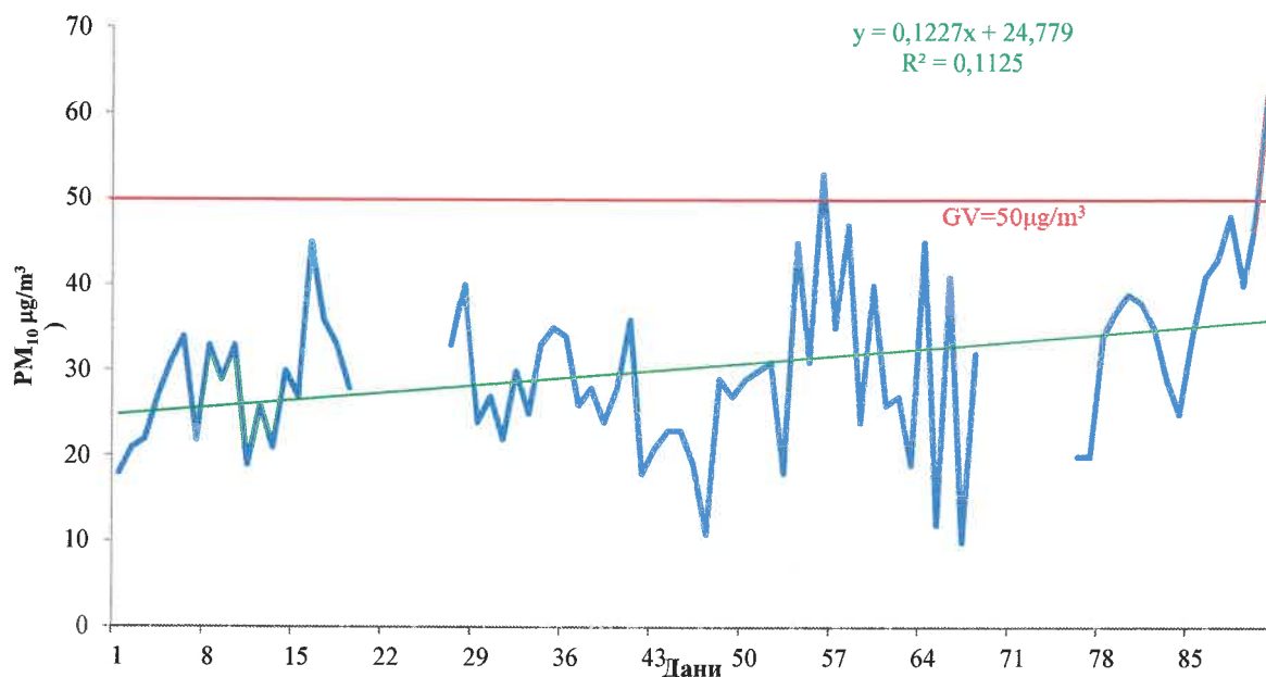
Графикон 5. PM_{10} у ваздуху амбијента на мерном месту Стрелиште, Панчево; II квартал 2026; Тренд дневних концентрација PM_{10}
