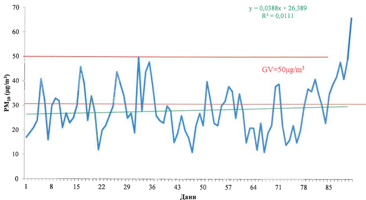
Графикон 6. PM_{10} у ваздуху амбијента на мерном месту Нова Миса, Панчево; II квартал 2026; Тренд дневних концентрација PM_{10}
