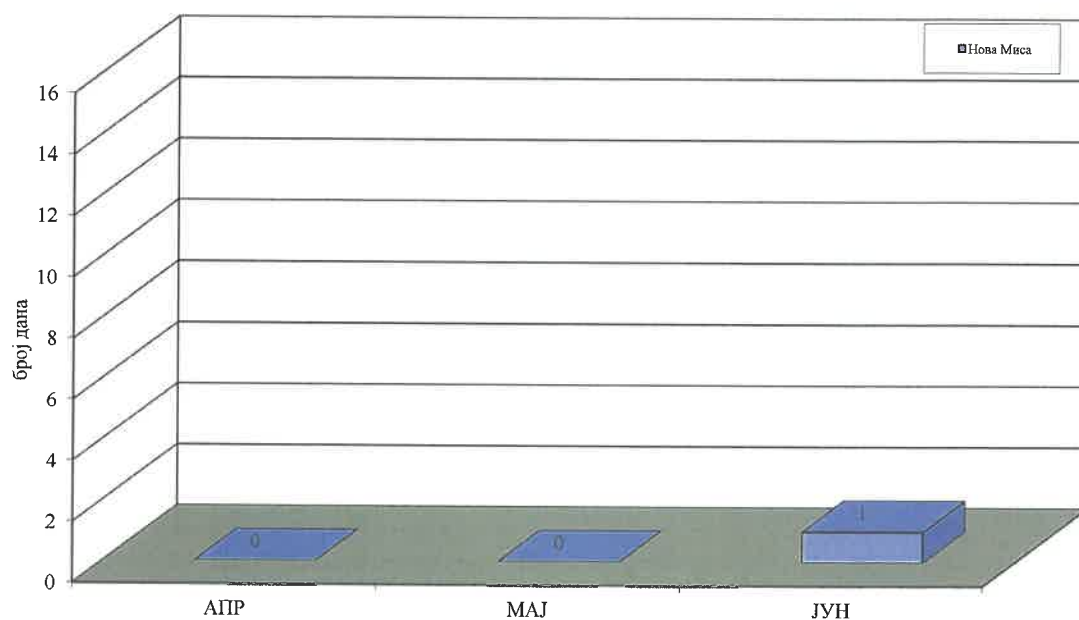
Графикон 4. PM_{10} у ваздуху амбијента на мерном месту Нова Миса, Панчево; II квартал 2026. Број дана са концентрацијама PM_{10} изнад GV
