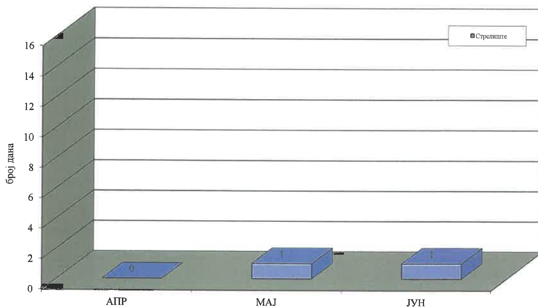
Графикон 3. PM_{10} у ваздуху амбијента на мерном месту Стрелиште, Панчево; II квартал 2026. Број дана са концентрацијама PM_{10} изнад GV
