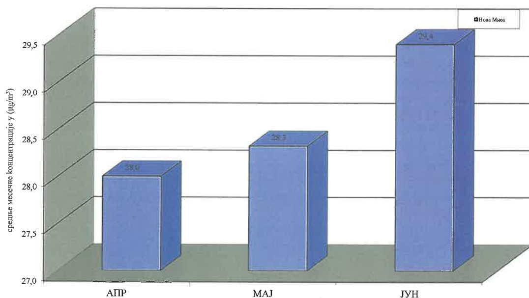
Графикон 2. PM 10 у ваздуху амбијента на мерном месту Нова Миса, Панчево; II квартал 2026. Дистрибуција средњих месечних концентрација
