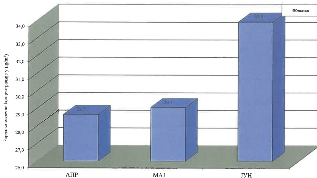
Графикон 1. PM 10 у ваздуху амбијента на мерном месту Стрелиште, Панчево; II квартал 2026. Дистрибуција средњих месечних концентрација
