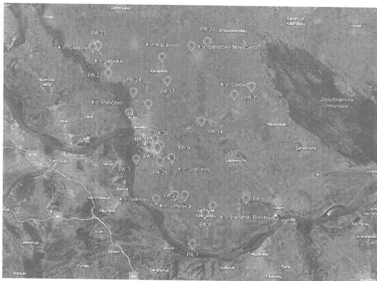
Slika 1. Zbimi prikaz lokacija uzorkovanja zemljišta na teritoriji Pančeva tokom I kampanje
