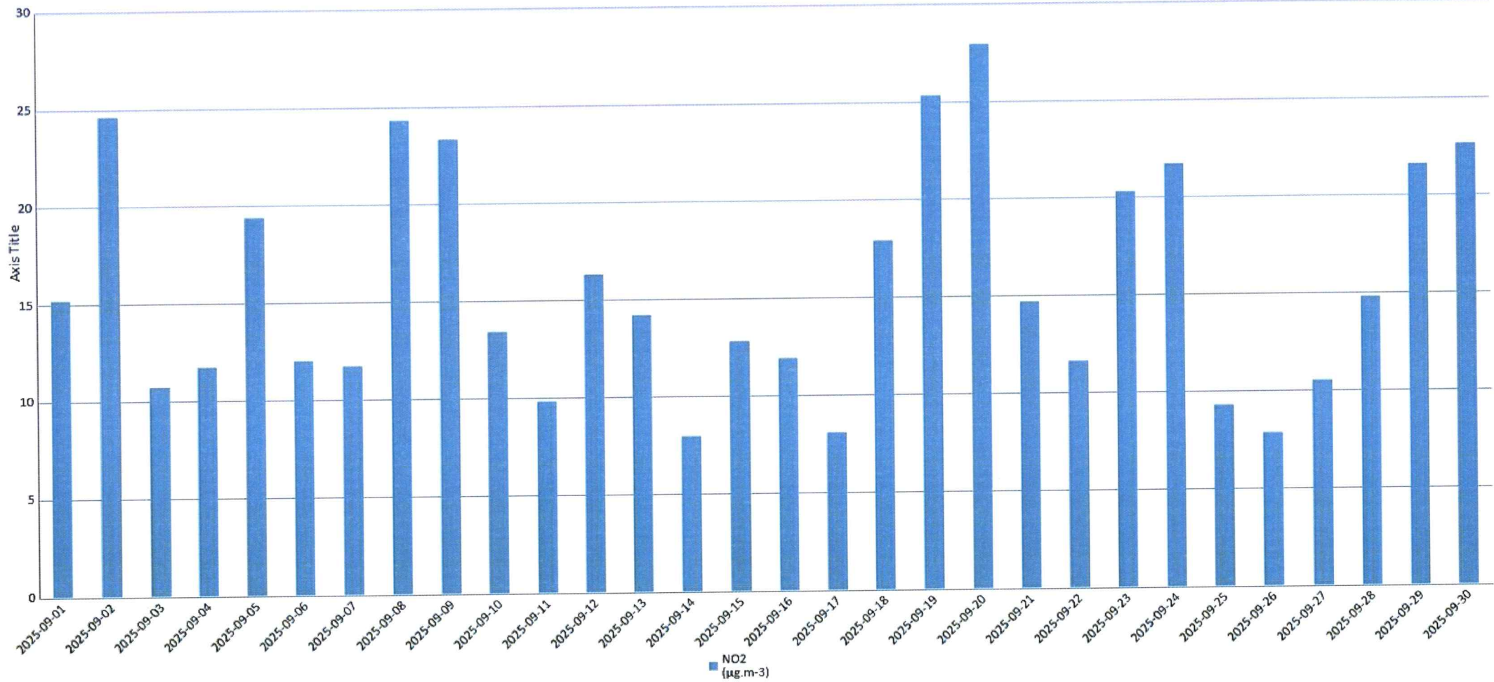
Старчево - NO 2
