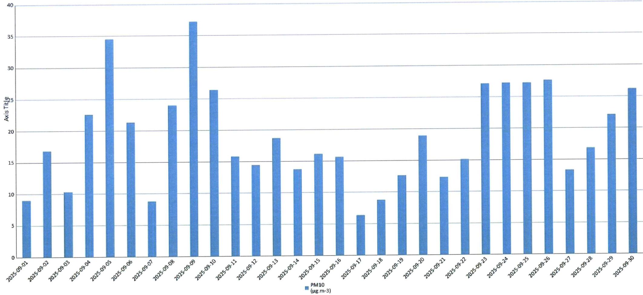
Војловица - PM10
