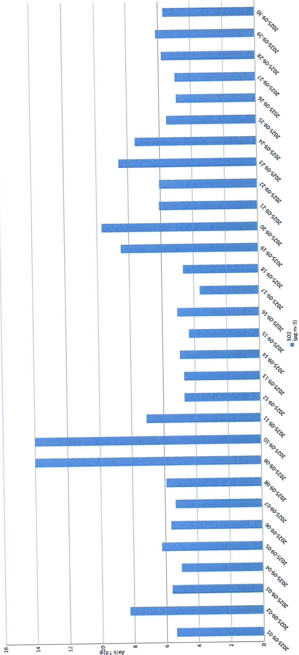
Старчево - SO 2
