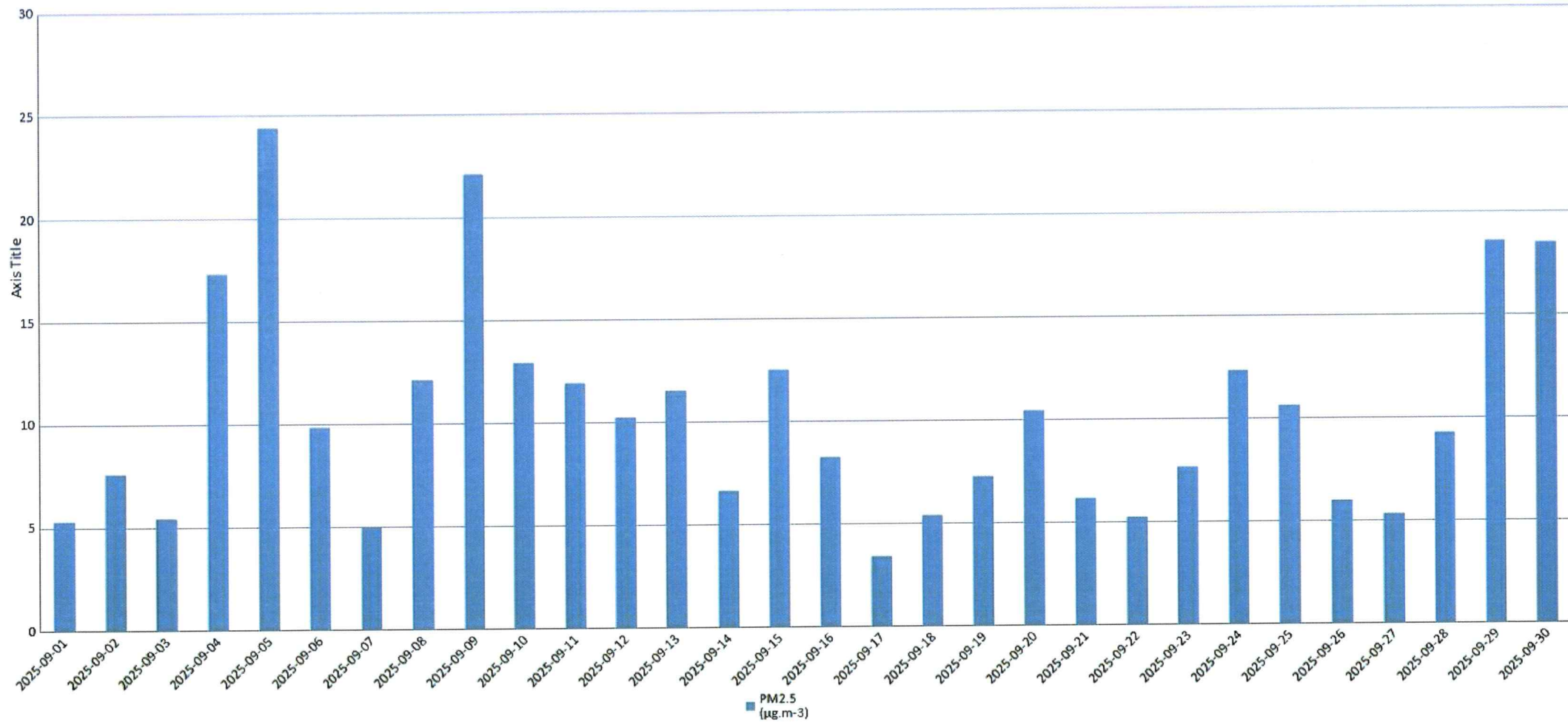
Војловица - PM2,5
