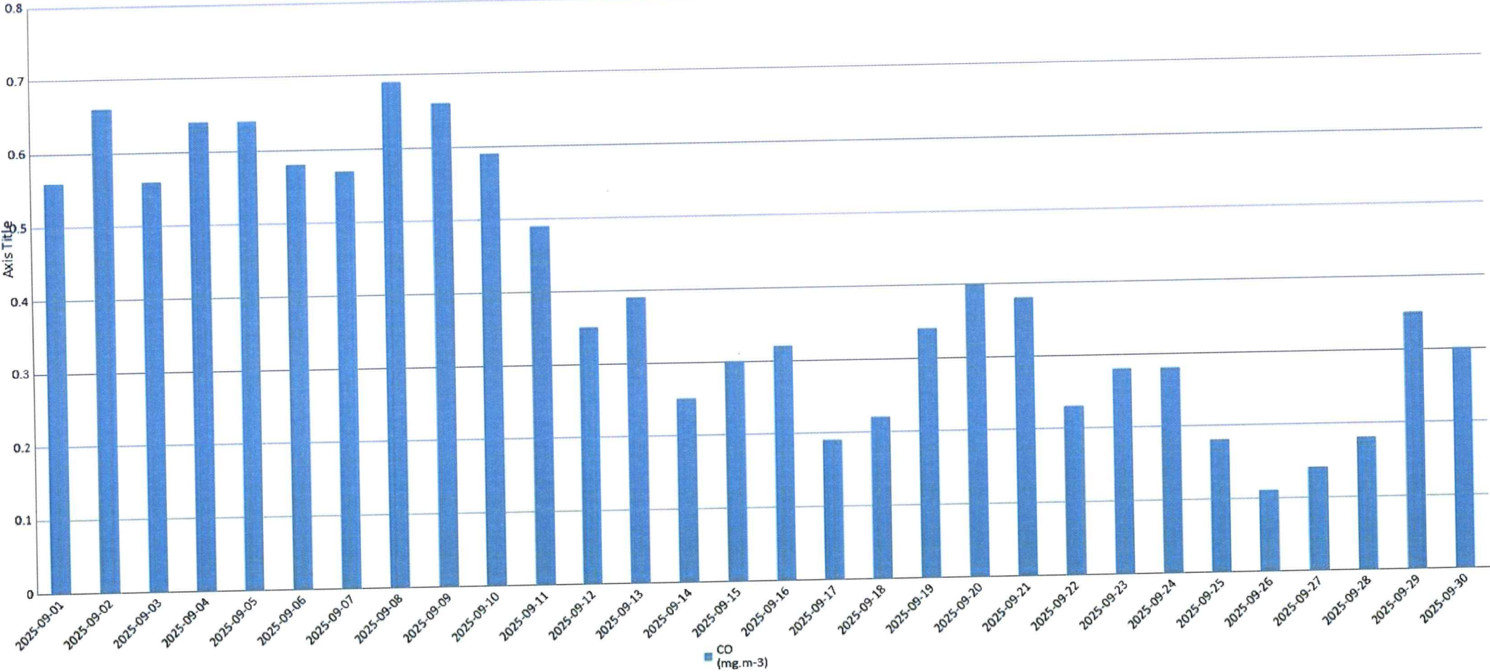
Старчево - CO
