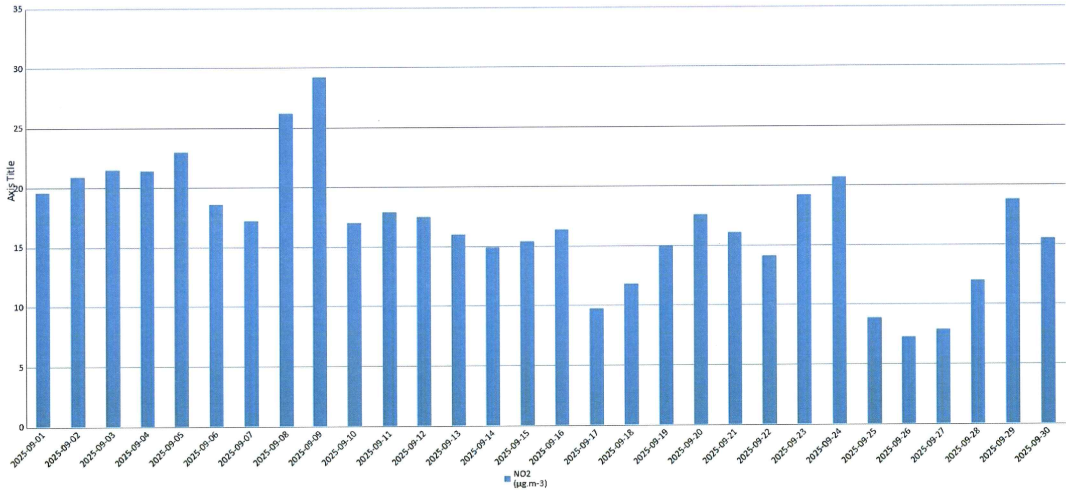
Војловица - NO 2
