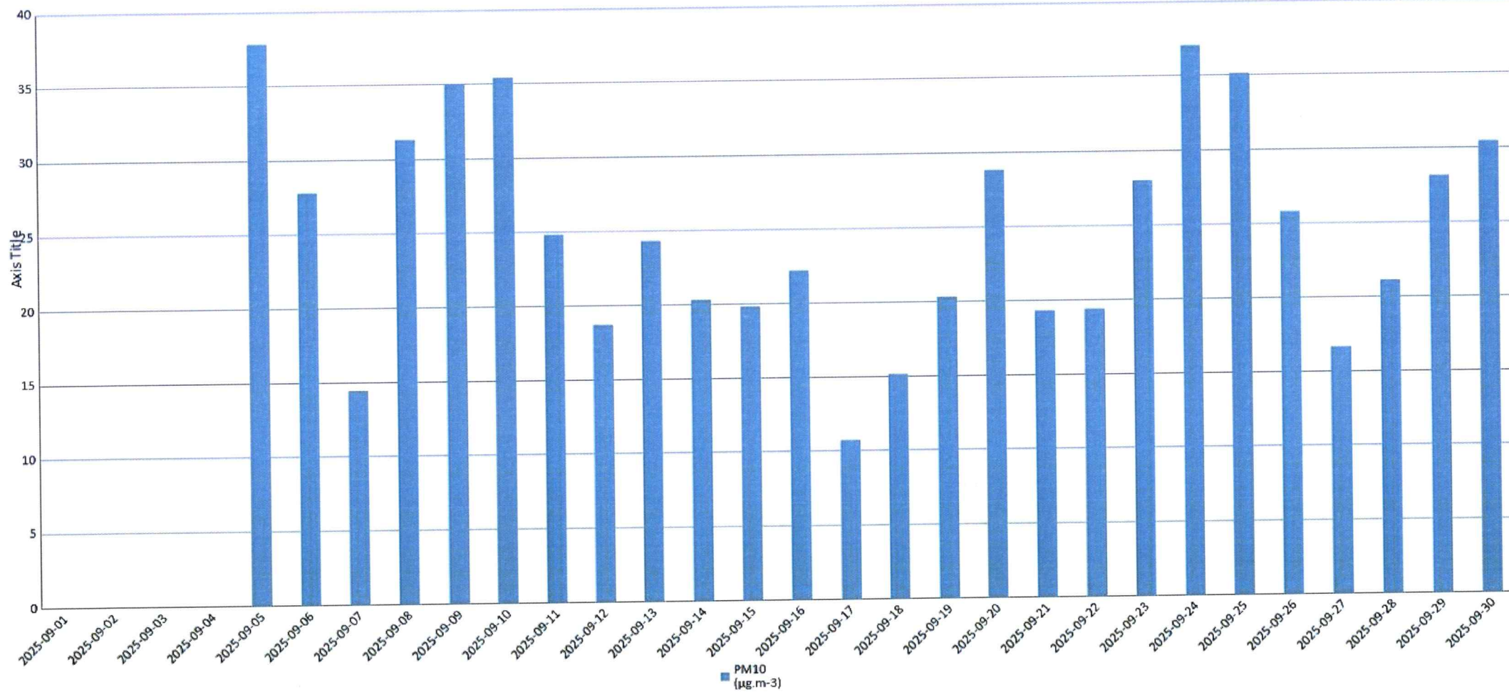
Старчево - PM10
