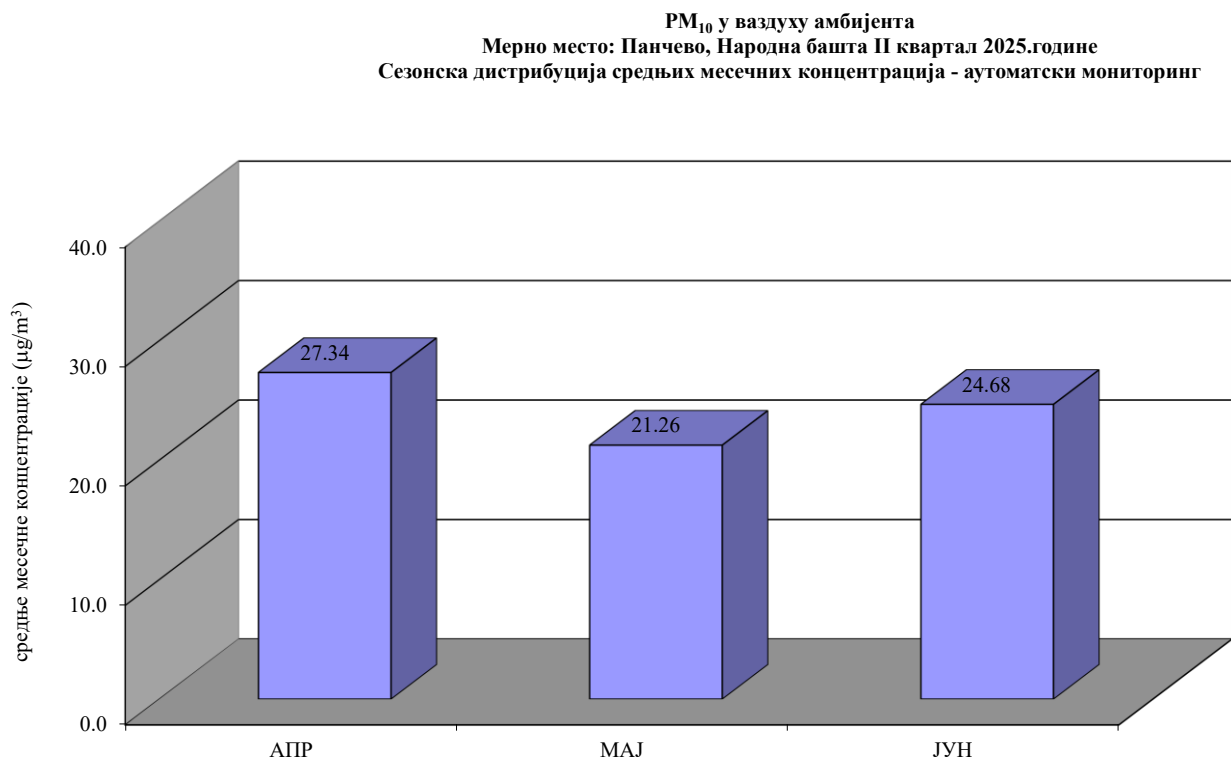
Графикон 1. Средње месечне концентрације PM 10 на мерном месту Народна башта, Панчево у периоду април-јун 2025.
