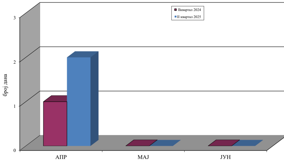
Графикон 9. Месечна дистрибуција броја дана са концентрацијама изнад граничне вредности за PM 10 на мерном месту Народна башта, Панчево - упоредни приказ април-јун 2024. и април-јун 2025.
