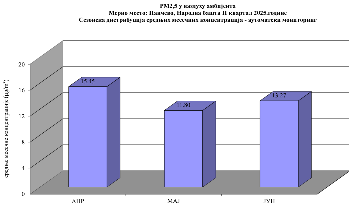
Графикон 2. Средње месечне концентрације PM 2,5 на мерном месту Народна башта, Панчево у периоду април-јун 2025.
