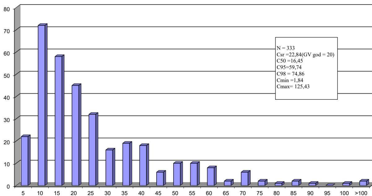
График 2. Дистрибуција релативних фреквенција PM 2,5
