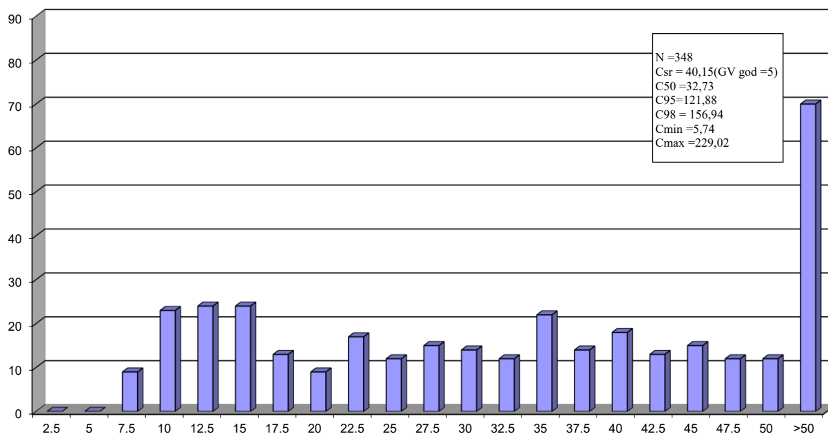
График 7. Дистрибуција релативних фреквенција ксилена
