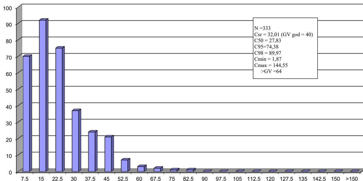
График 1. Дистрибуција релативних фреквенција PM 10
