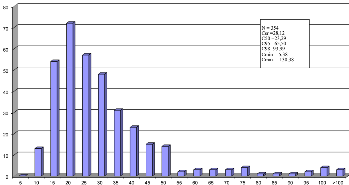
График 4. Дистрибуција релативних фреквенција азотних оксида
