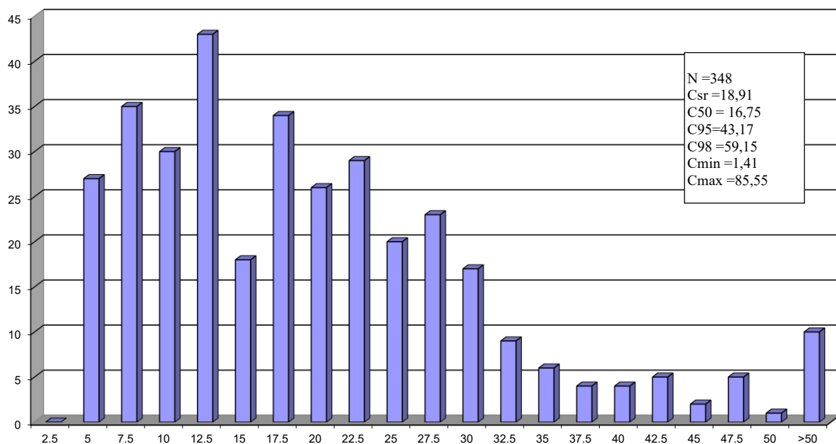
График 6. Дистрибуција релативних фреквенција толуена
