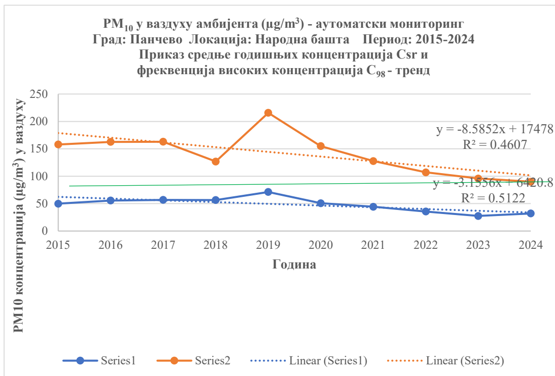
График 15. Средње годишње концентрације и фреквенција високих концентрација C 98 за PM 10
