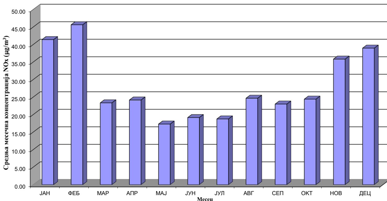
График 11. Средње месечне концентрације азотних оксида
