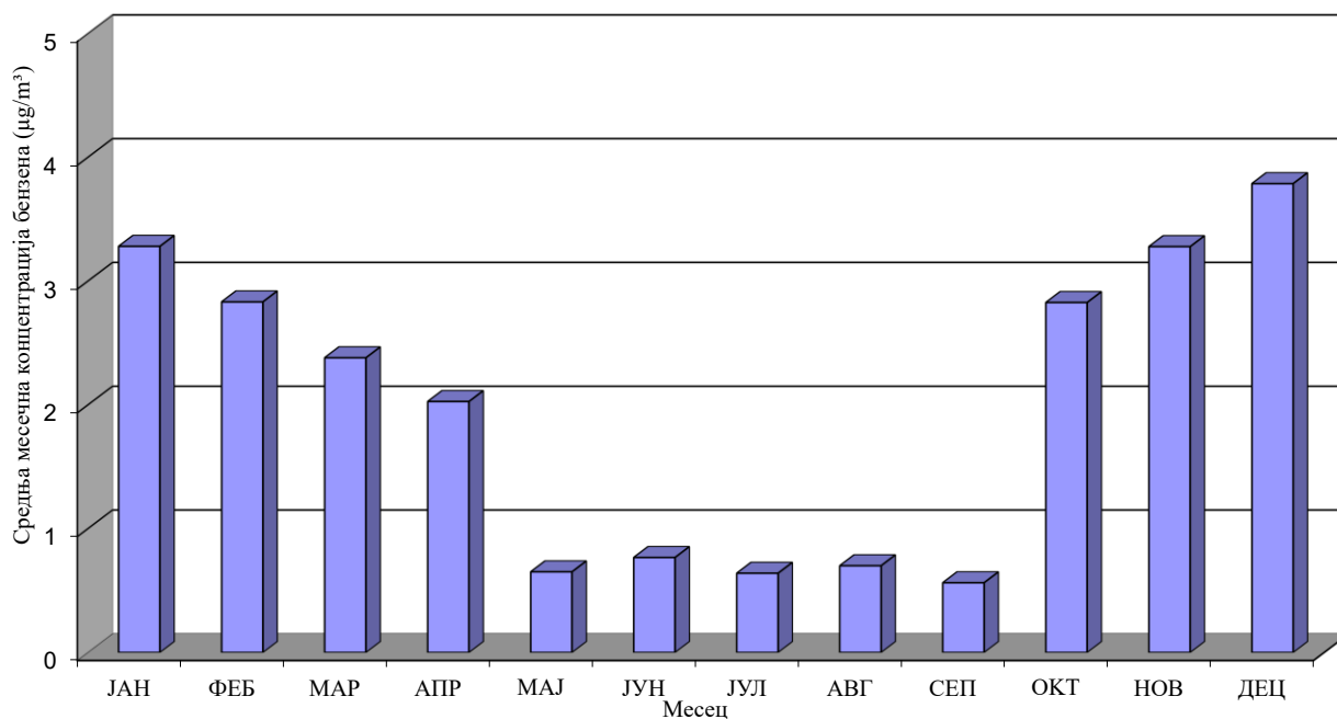
График 12. Средње месечне концентрације бензена
