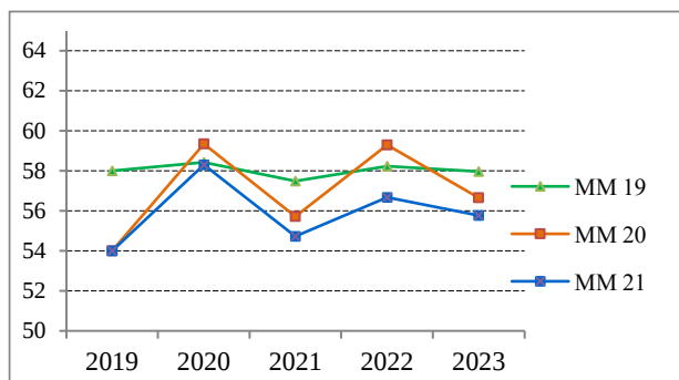
Графикон 30. Вредности L_{den} у периоду 2019 – 2023.год. на ММ 19,20 и 21
