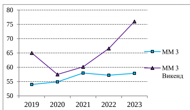
Графикон 22. Вредности L_{den} у периоду 2019 – 2023. год. на ММ 3 (радни дан и викенд)
