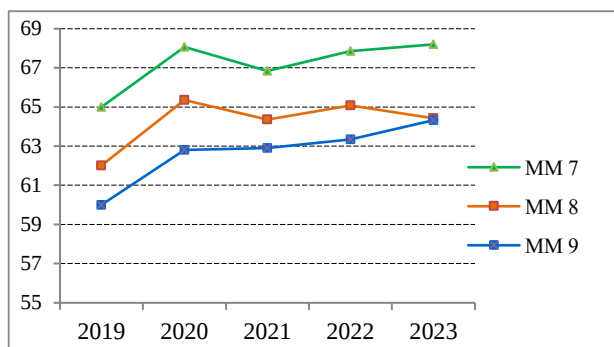
Графикон 26. Вредности L_{den} у периоду 2019 – 2023.год. на ММ 7, 8 и 9
