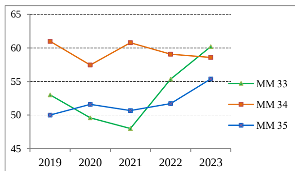
Графикон 37. Вредности L_{den} у периоду 2019 – 2023.год. на ММ 33,34 и 35
