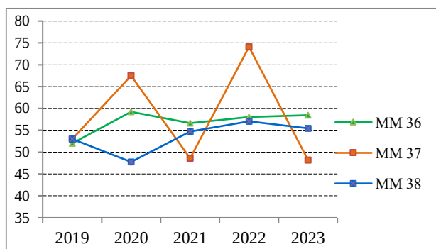
Графикон 38. Вредности L_{den} у периоду 2019 – 2023.год. на ММ 36,37 и 38
