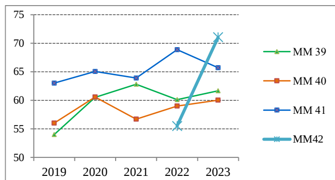
Графикон 39. Вредности L_{den} у периоду 2019 – 2023.год. на ММ 39,40,41 и 42
