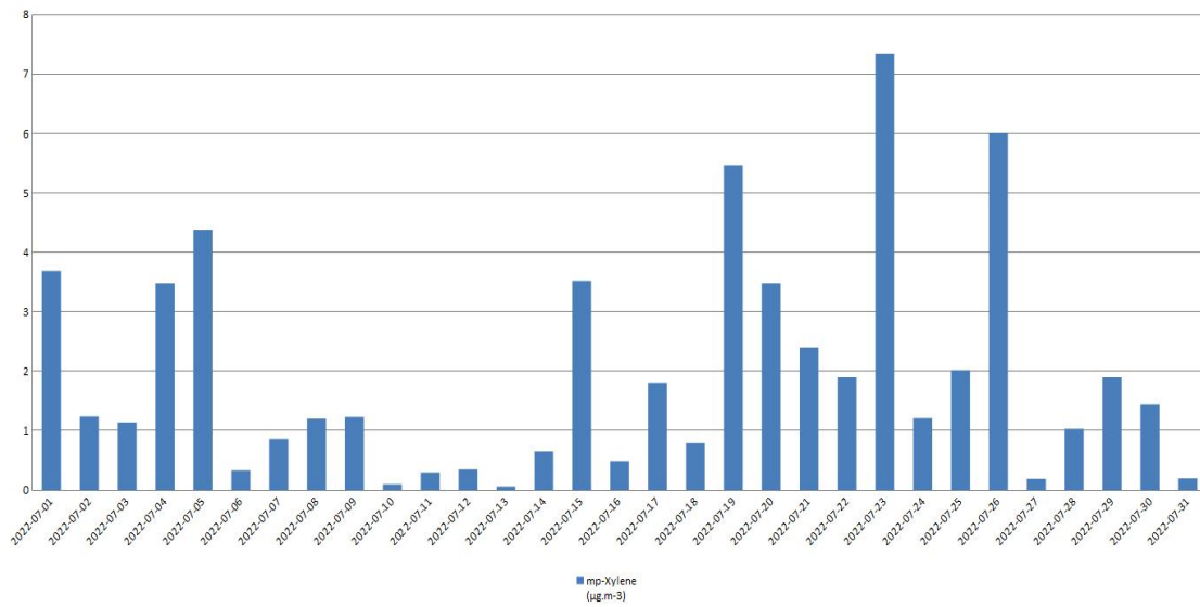
Војловица - Ксилен
