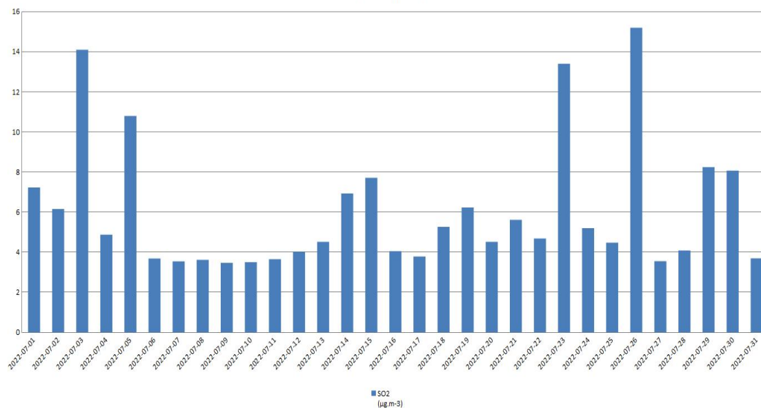
Војловица - SO 2
