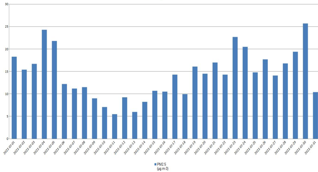
Војловица - PM2.5
