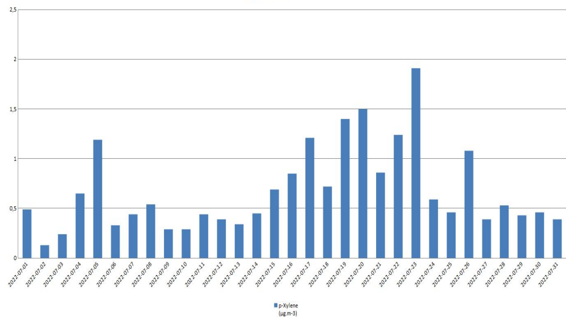
Цара Душана - Ксилен
