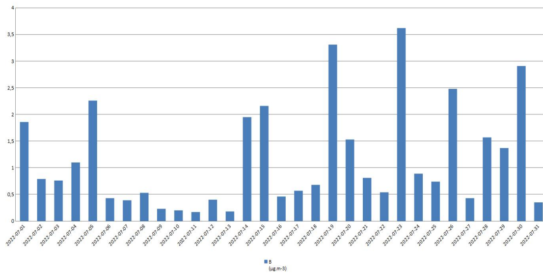
Војловица - Бензен
