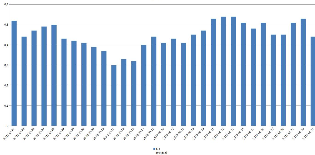
Старчево - CO
