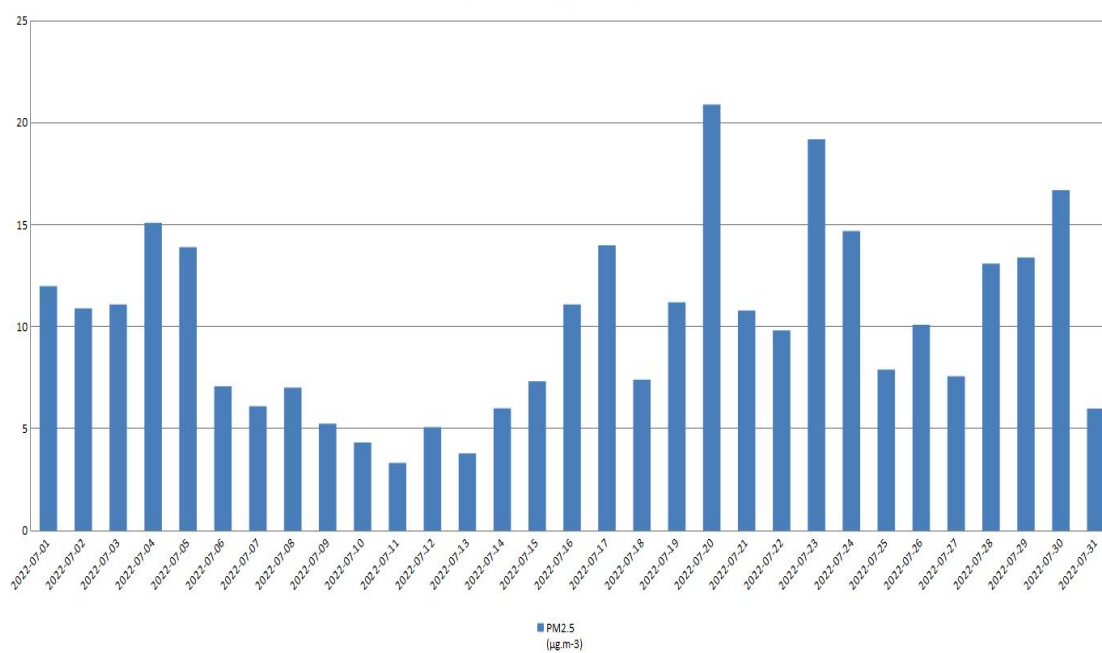
Ватрогасни дом - PM2.5
