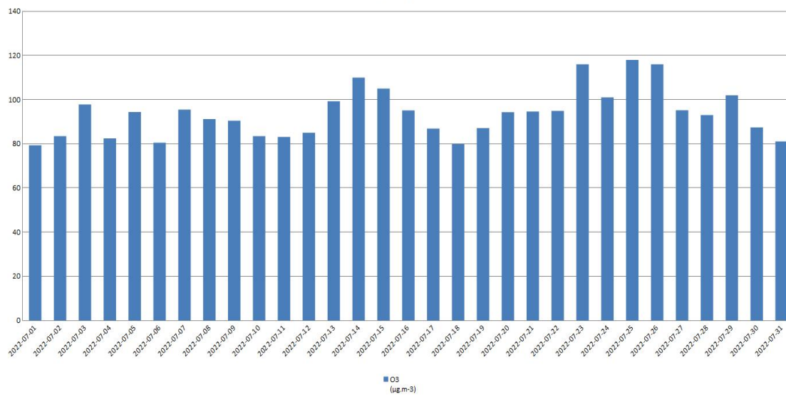
Старчево - O3
