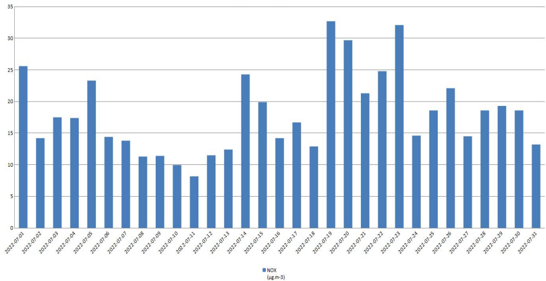
Ватрогасни дом - NOx
