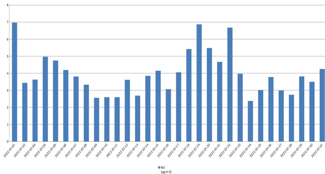
Старчево - NO
