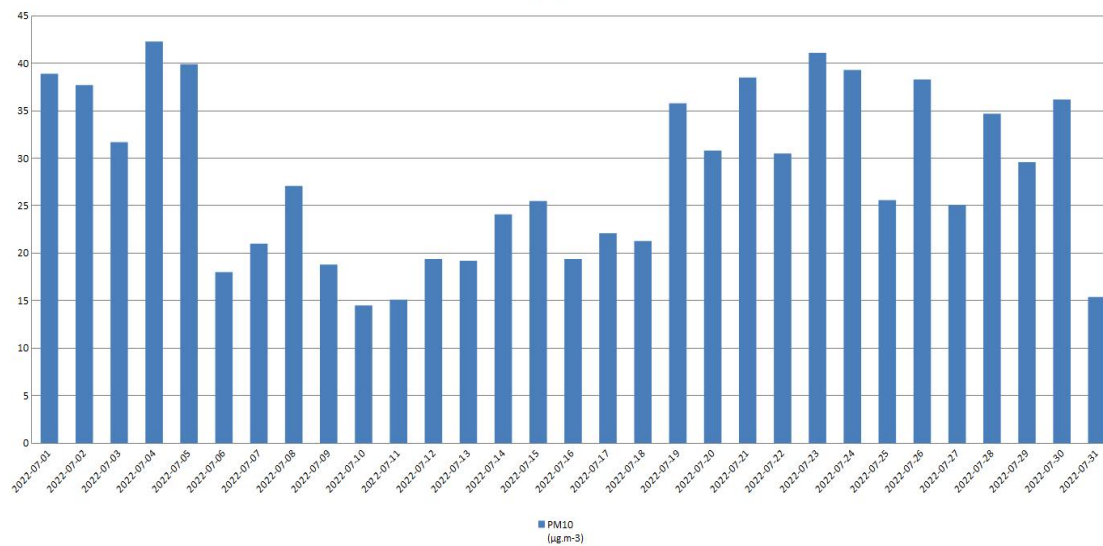
Војловица - PM 10
