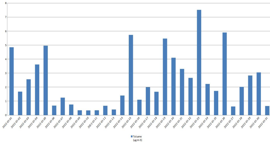
Војловица - Толуен
