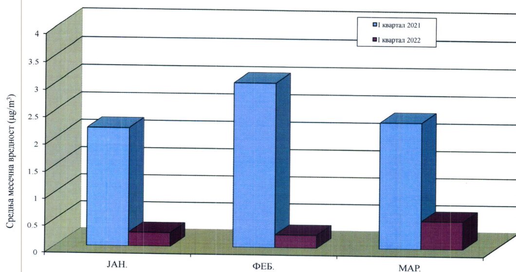
Графикон 11. Дистрибуција просечних месечних концентрација амонијака на мерном месту Народна башта, Панчево - упоредни приказ јануар – март 2021. и јануар – март 2022.
