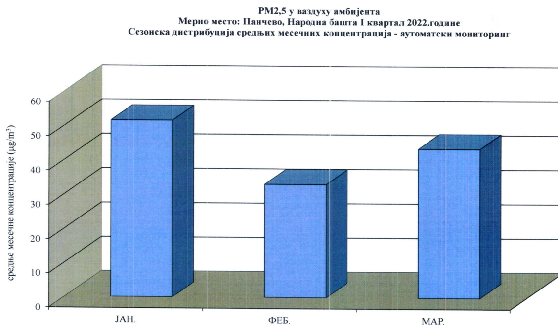
Графикон 2. Средње месечне концентрације PM 2,5 на мерном месту Народна башта, Панчево у периоду јануар – март 2022.
