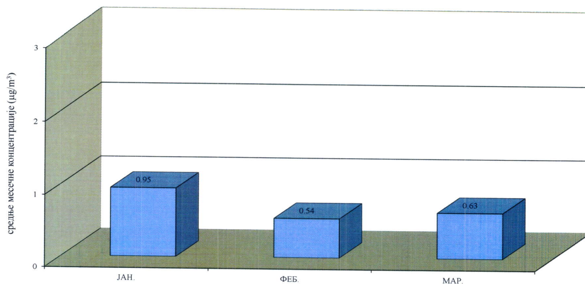
Графикон 5. Средње месечне концентрације бензена на мерном месту Народна башта, Панчево у периоду јануар – март 2022.
