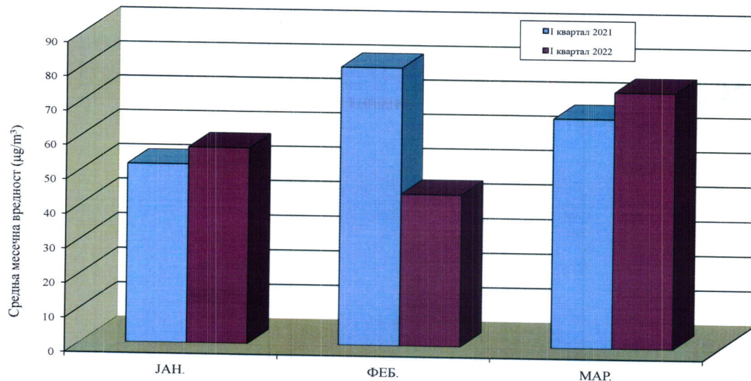
Графикон 10. Дистрибуција просечних месечних концентрација PM 10 на мерном месту Народна башта, Панчево - упоредни приказ јануар – март 2021. и јануар – март 2022.
