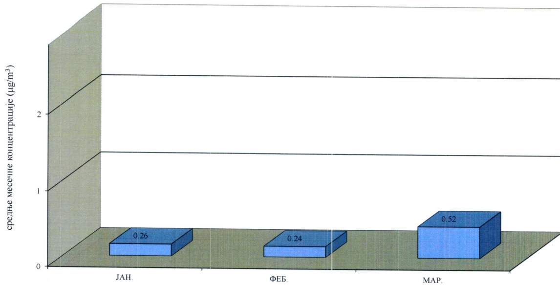
Графикон 3. Средње месечне концентрације амонијака на мерном месту Народна башта, Панчево у периоду јануар – март 2022.
