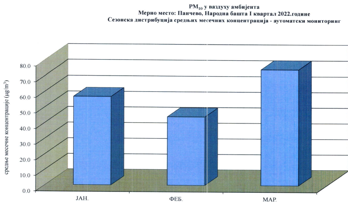
Графикон 1. Средње месечне концентрације PM 10 на мерном месту Народна башта, Панчево у периоду јануар – март 2022.
