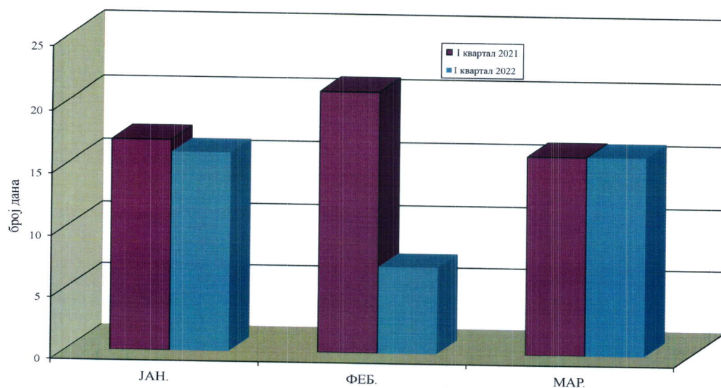
Графикон 9. Месечна дистрибуција броја дана са концентрацијама изнад граничне вредности за PM 10 на мерном месту Народна башта, Панчево - упоредни приказ јануар – март 2021. и јануар – март 2022.
