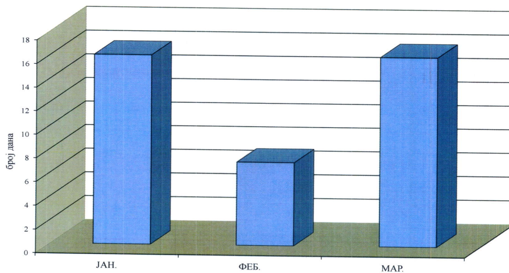
Графикон 8. Месечна дистрибуција броја дана са концентрацијама изнад граничне вредности за PM 10 на мерном месту Народна башта, Панчево у периоду јануар – март 2022.
