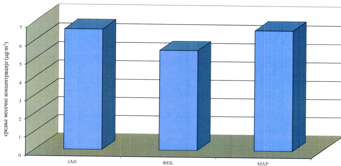
Графикон 7. Средње месечне концентрације ксилена на мерном месту Народна башта, Панчево у периоду јануар – март 2022.
