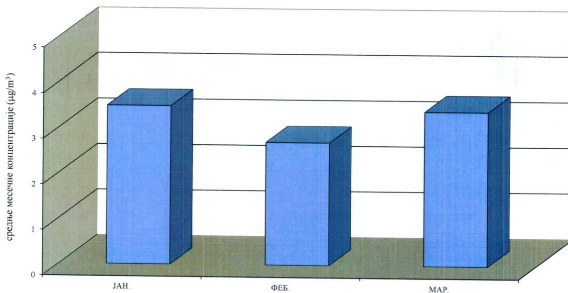
Графикон 6. Средње месечне концентрације толуена на мерном месту Народна башта, Панчево у периоду јануар – март 2022.
