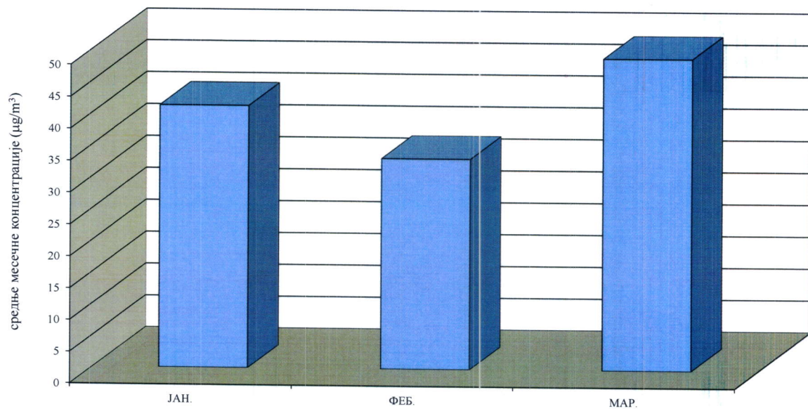
Графикон 4. Средње месечне концентрације азотних оксида на мерном месту Народна башта, Панчево у периоду јануар – март 2022.
