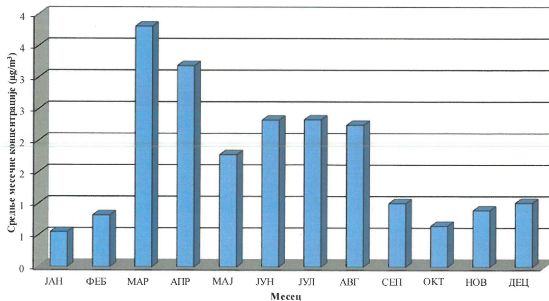
Бензен у ваздуху амбијента Мерно место: Народна башта, Панчево, 2021 година Дистрибуција средњих месечних концентрација ( \mu\text{g}/\text{m}^3 ) -аутоматски мониторинг-
