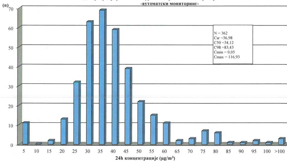
NOx у ваздуху амбијента Мерно место: Народна башта, Панчево, 2021. година Дистрибуција релативних фреквенција 24h концентрација -аутоматски мониторинг-
