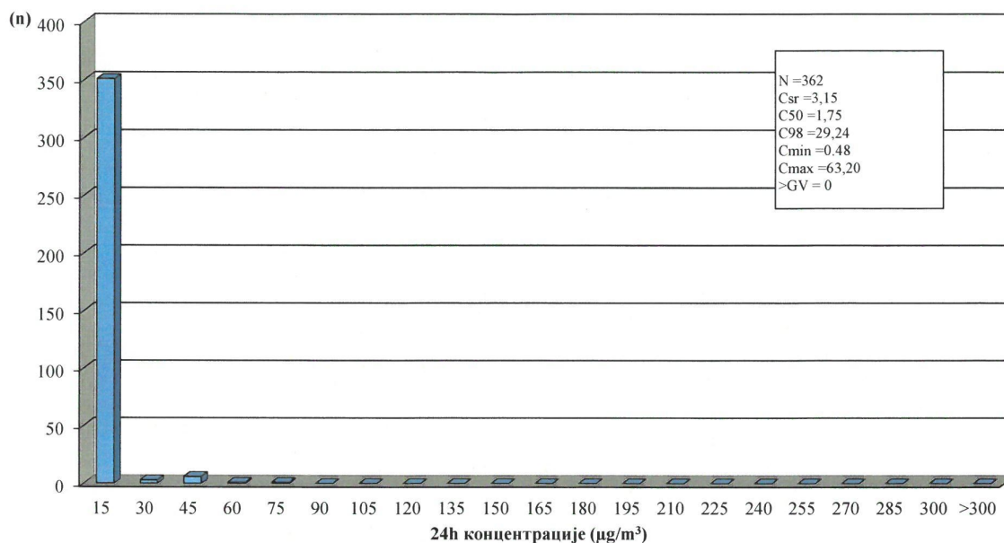
Амонијак у ваздуху амбијента Мерно место: Народна башта, Панчево, 2021. година Дистрибуција релативних фреквенција 24h концентрација -аутоматски мониторинг-
