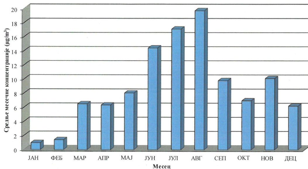
Толуен у ваздуху амбијента Мерно место: Народна башга, Панчево, 2021 година Дистрибуција средњих месечних концентрација ( \mu\text{g}/\text{m}^3 ) -аутоматски мониторинг-
