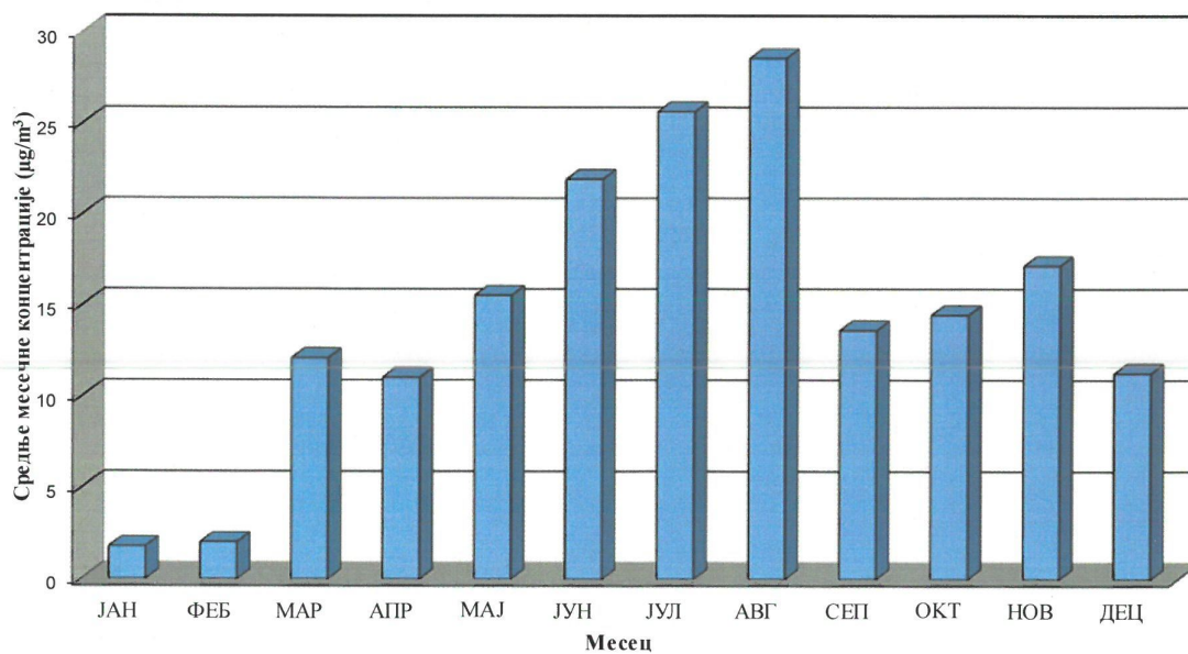
Ксилен у ваздуху амбијента Мерно место: Народна башга, Панчево, 2021 година Дистрибуција средњих месечних концентрација ( \mu\text{g}/\text{m}^3 ) -аутоматски мониторинг-
