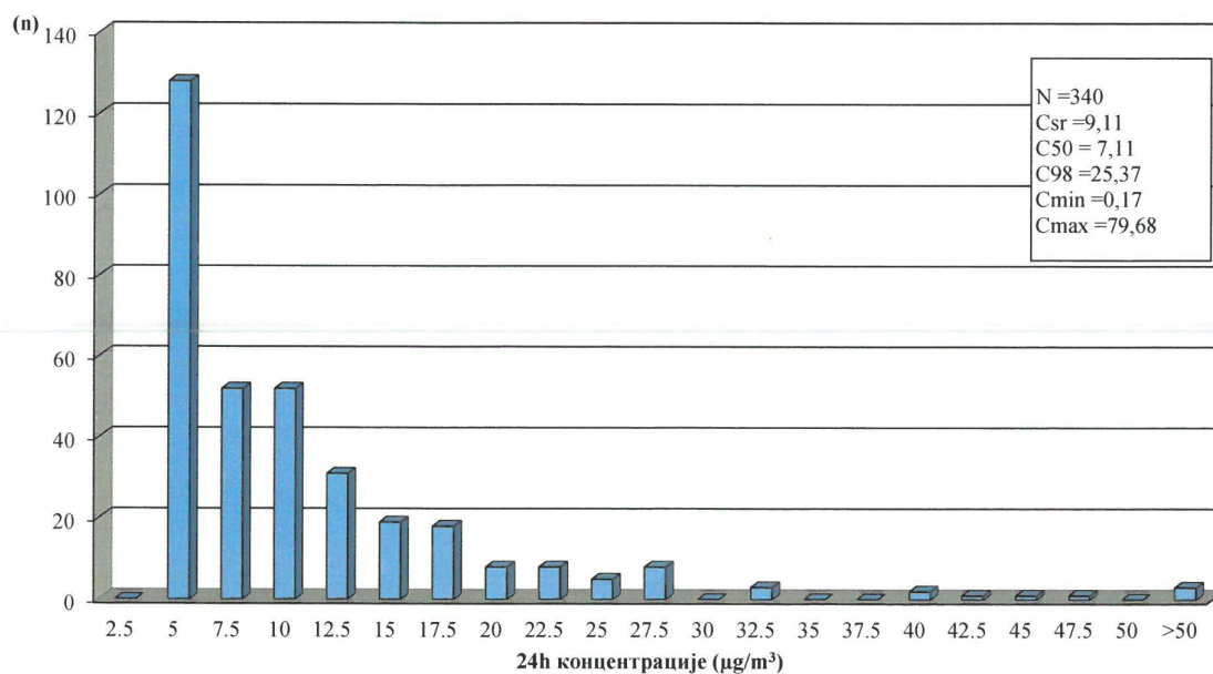
Толуен у ваздуху амбијента Мерно место: Народна башта, Панчево, 2021. година Дистрибуција релативних фреквенција 24h концентрација -аутоматски мониторинг-
