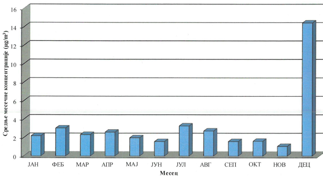
Амонијак у ваздуху амбијента Мерно место: Народна башта, Панчево, 2021 година Дистрибуција средњих месечних концентрација ( \mu\text{g}/\text{m}^3 ) -аутоматски мониторинг-
