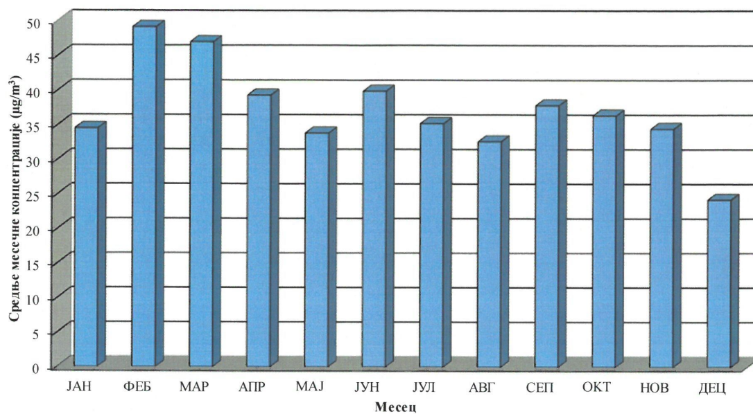
NOx у ваздуху амбијента Мерно место: Народна башта, Панчево 2021 година Дистрибуција средњих месечних концентрација ( \mu\text{g}/\text{m}^3 ) -аутоматски мониторинг-
