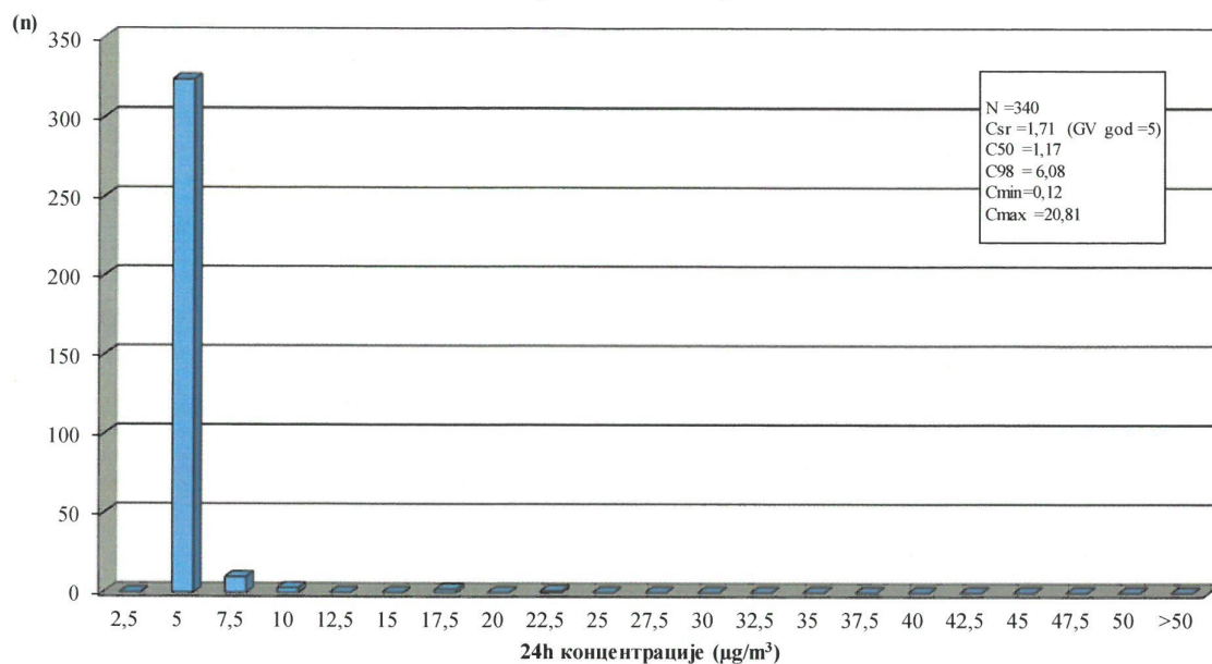
Бензен у ваздуху амбијента Мерно место: Народна башта, Панчево 2021. година Дистрибуција релативних фреквенција 24h концентрација -аутоматски мониторинг-
