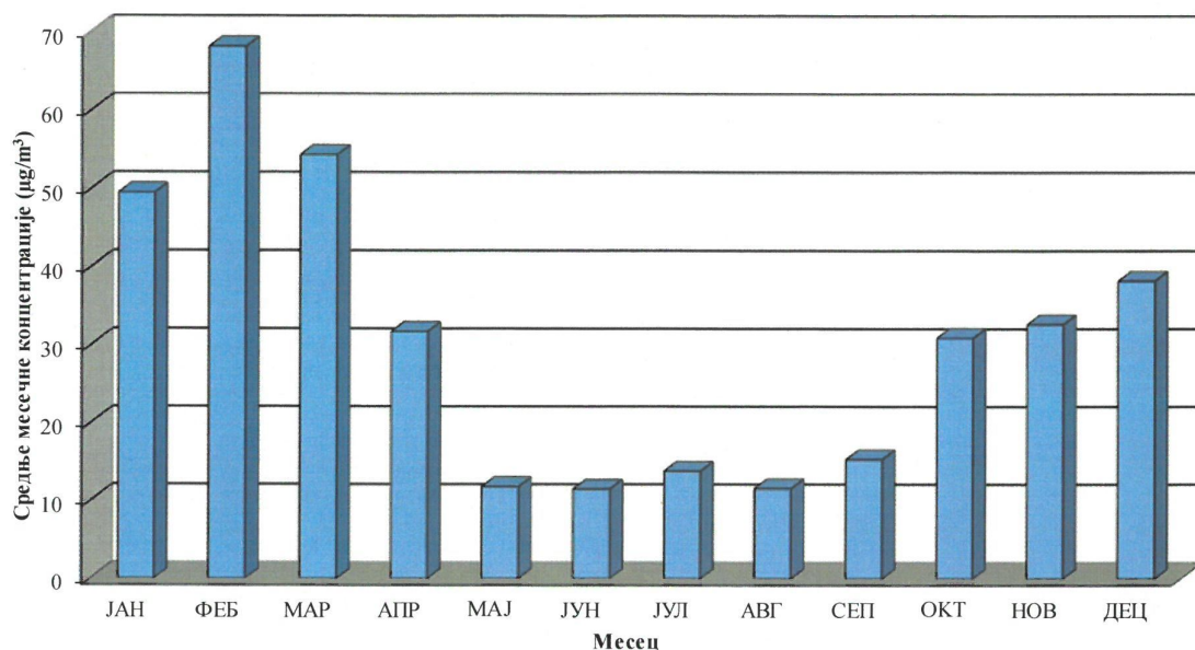
PM 2,5 у ваздуху амбијента Мерно место: Народна башта, Панчево, 2021 година Дистрибуција средњих месечних концентрација ( \mu\text{g}/\text{m}^3 ) -аутоматски мониторинг-
