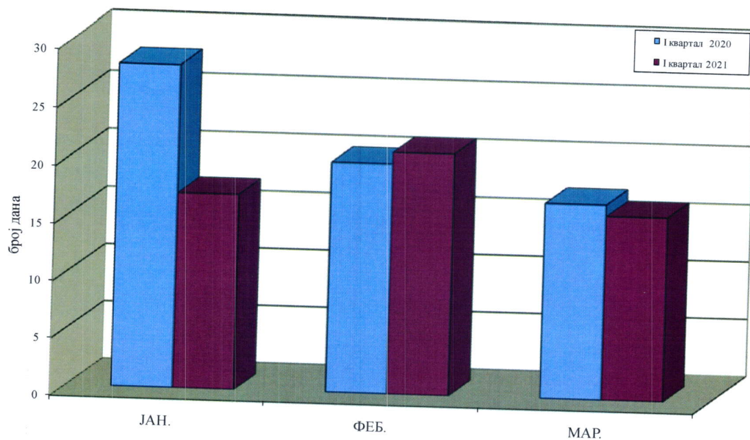
PM 10 У ВАЗДУХУ АМБИЈЕНТА Мерно место: Панчево, Народна башта Упоредни приказ броја дана са концентрацијама изнад GV I квартал 2020.-I квартал 2021.
