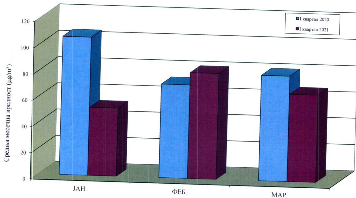
PM 10 У ВАЗДУХУ АМБИЈЕНТА Мерно место: Панчево, Народна башта Упоредни приказ просечних месечних концентрација I квартал 2020. - I квартал 2021.
