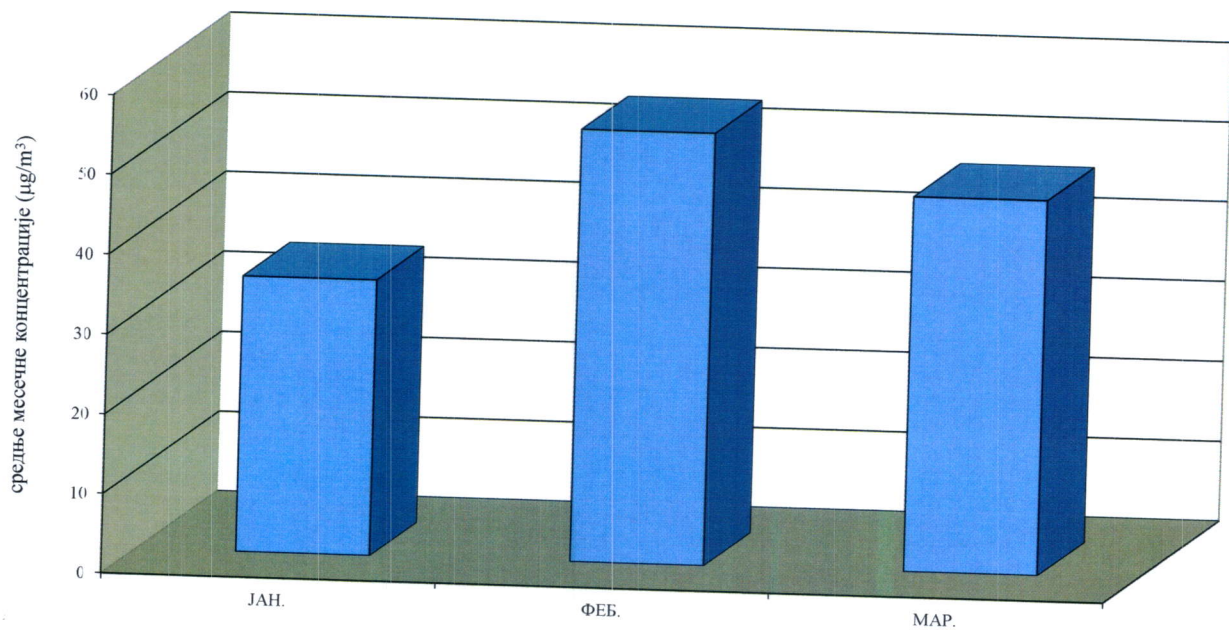
Азотни оксиди у ваздуху амбијента Мерно место: Панчево, Народна башта I квартал 2021.године Сезонска дистрибуција средњих месечних концентрација - аутоматски мониторинг
