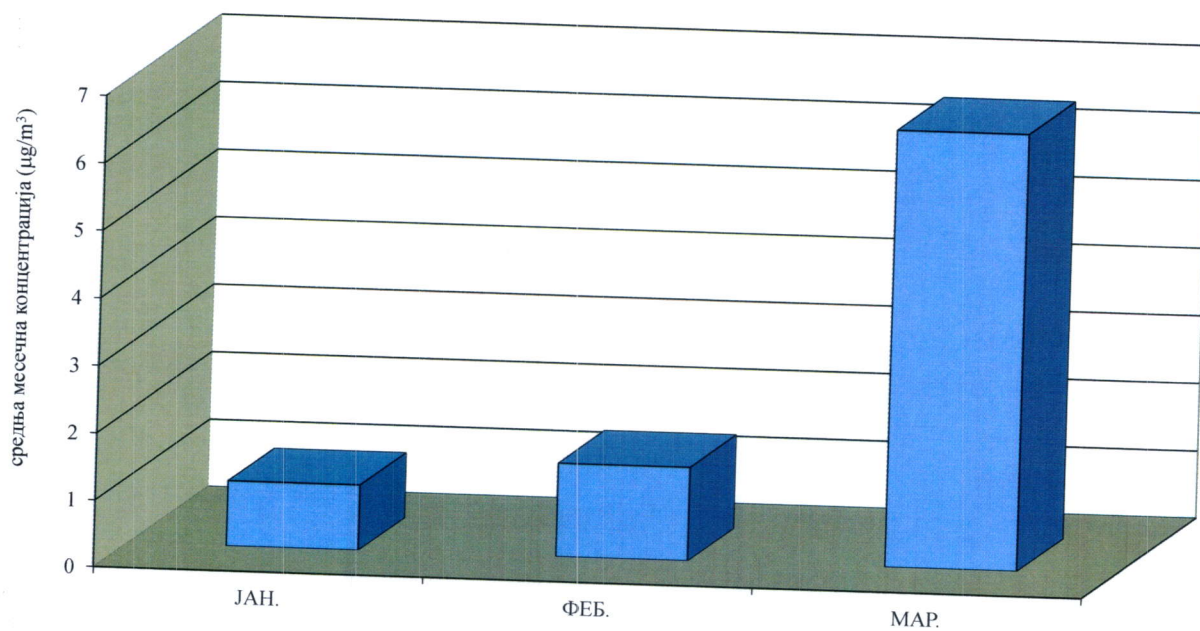
Толуен у ваздуху амбијента Мерно место: Панчево, Народна башта I квартал 2021.године Сезонска дистрибуција средњих месечних концентрација - аутоматски мониторинг
