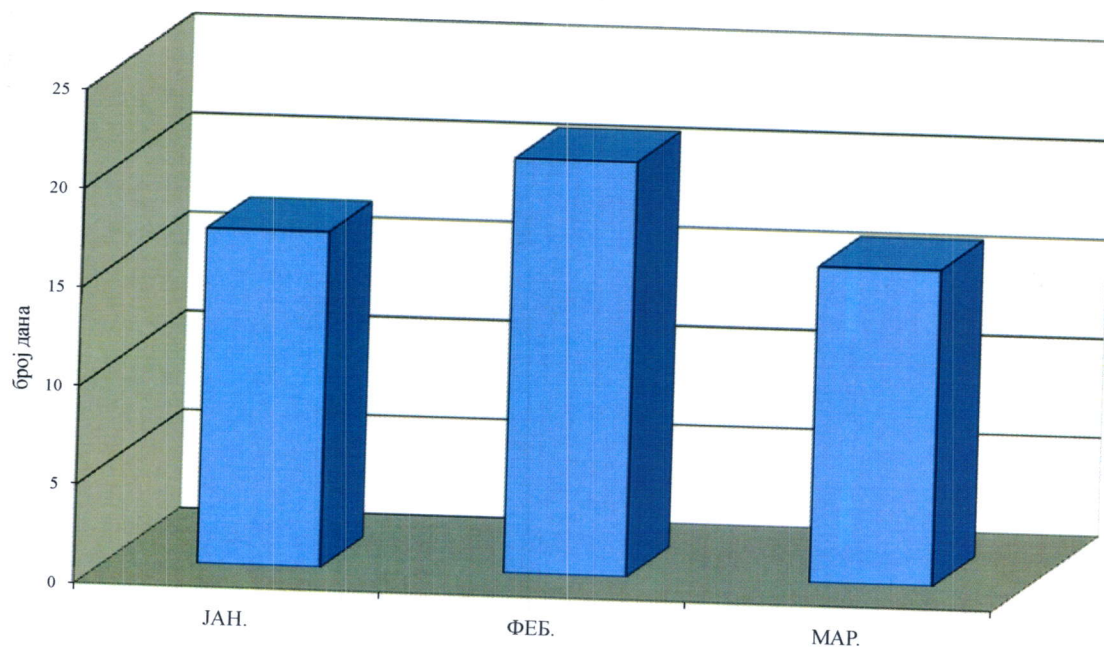
PM 10 У ВАЗДУХУ АМБИЈЕНТА Мерно место: Панчево, Народна башта Број дана са концентрацијама PM 10 изнад GV I квартал 2021.
