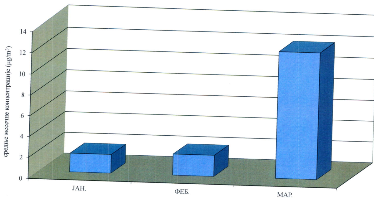
Бензен у ваздуху амбијента Мерно место: Панчево, Народна башта I квартал 2021.године Сезонска дистрибуција средњих месечних концентрација - аутоматски мониторинг
