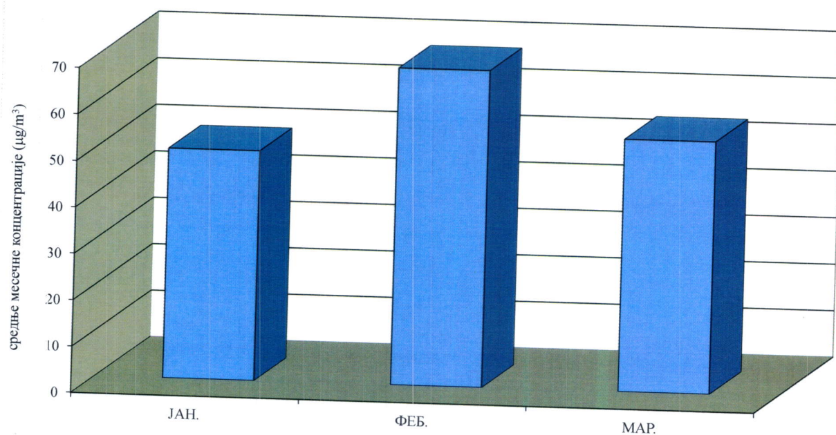
PM 2,5 у ваздуху амбијента Мерно место: Панчево, Народна башта I квартал 2021.године Сезонска дистрибуција средњих месечних концентрација - аутоматски мониторинг
