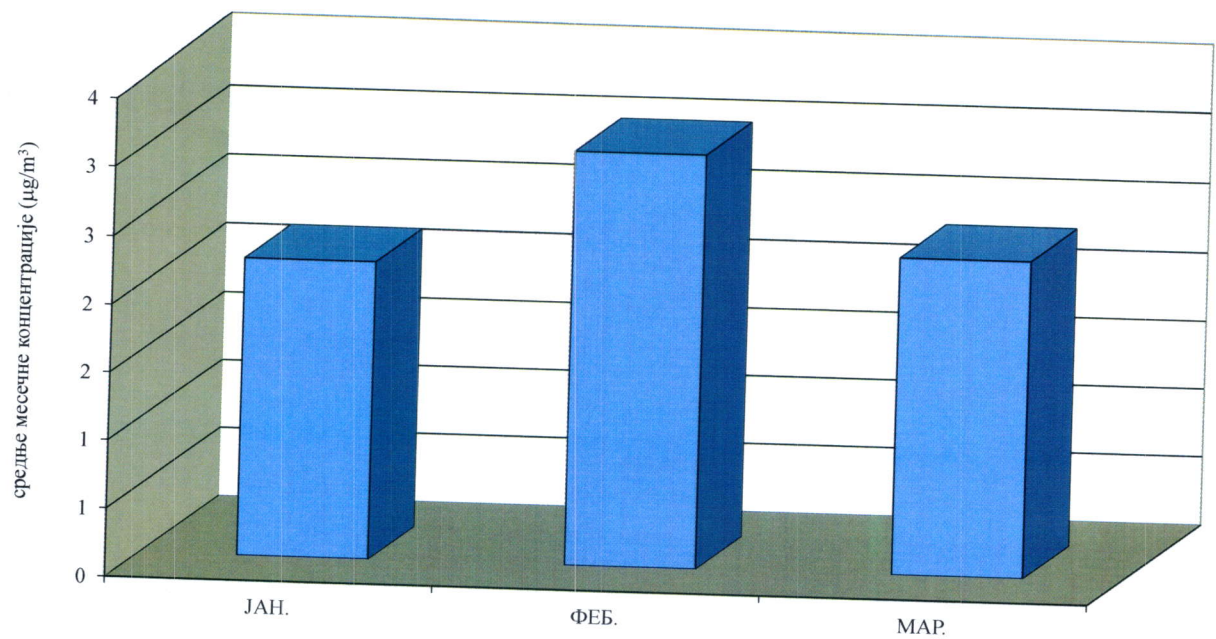
Амонијак у ваздуху амбијента Мерно место: Панчево, Народна башта I квартал 2021.године Сезонска дистрибуција средњих месечних концентрација - аутоматски мониторинг
