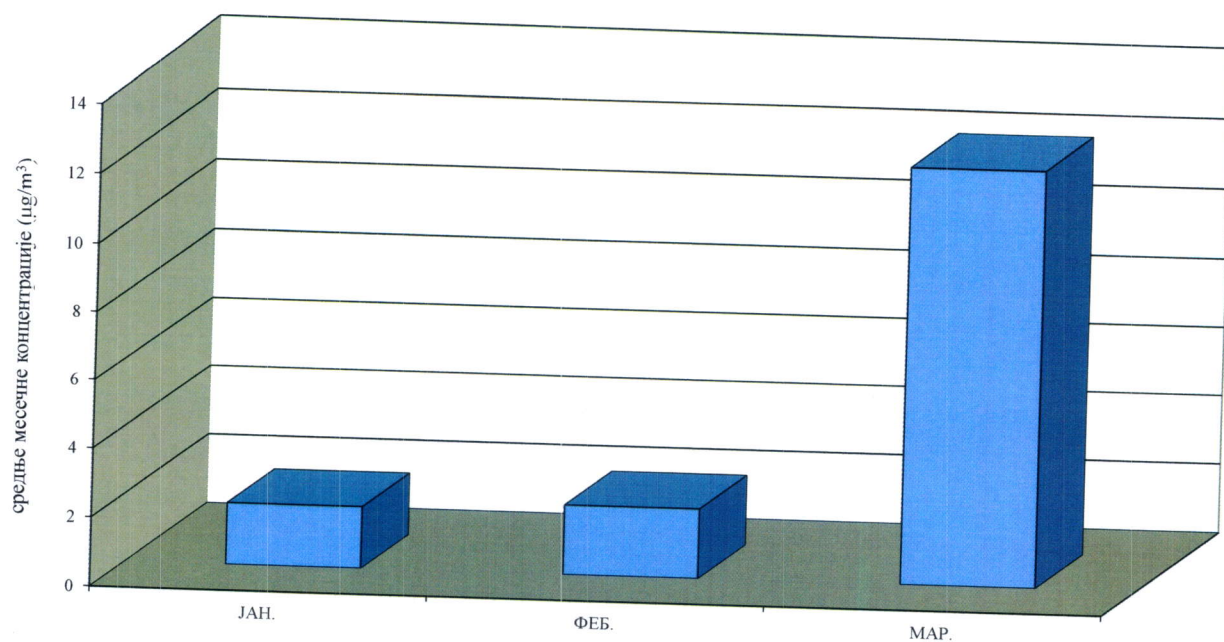
Ксилен у ваздуху амбијента Мерно место: Панчево, Народна башта I квартал 2021.године Сезонска дистрибуција средњих месечних концентрација - аутоматски мониторинг
