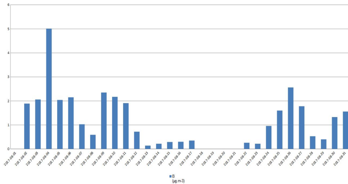
Војловица - бензен
