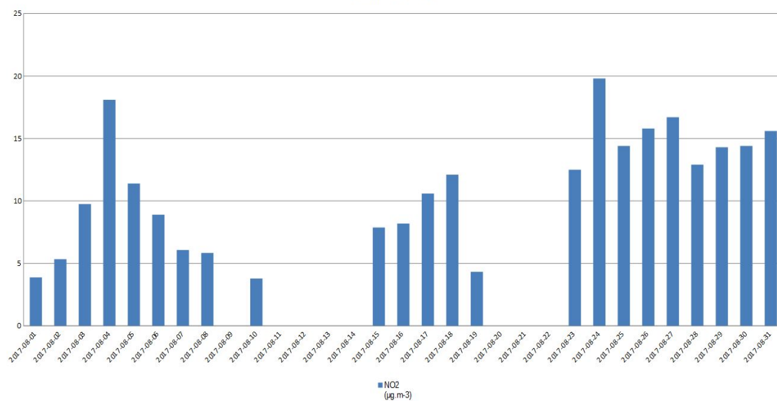
Старчево NO2
