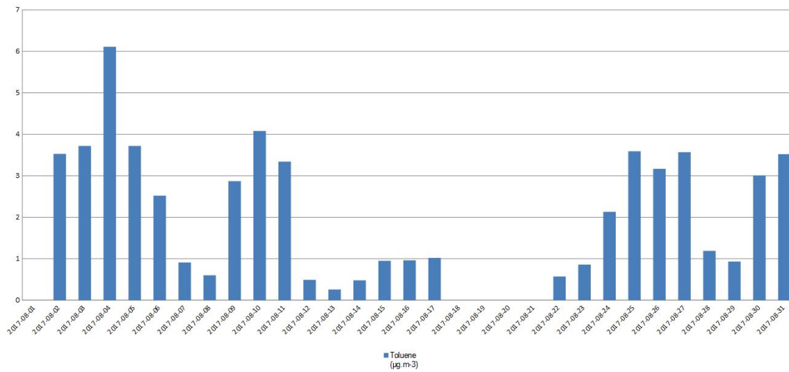
Војловица - толуен
