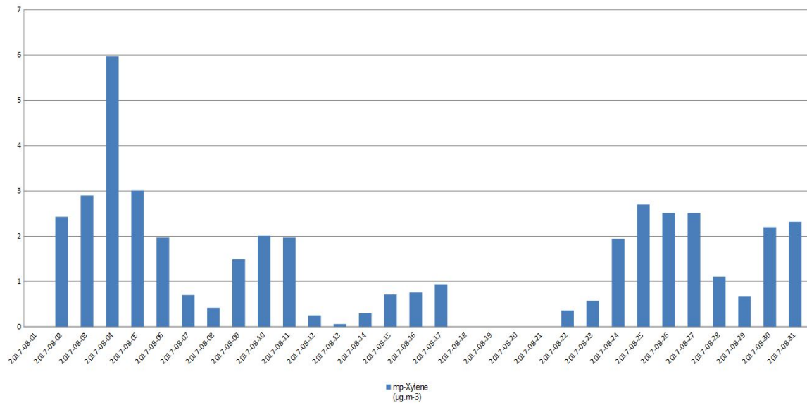
Војловица - ксилен
