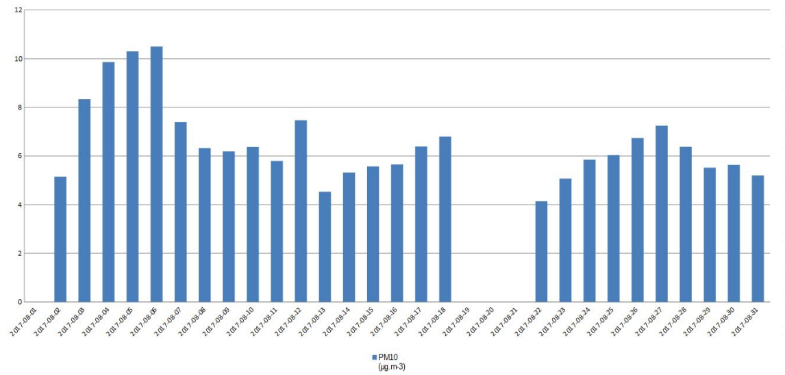
Војловица PM10
