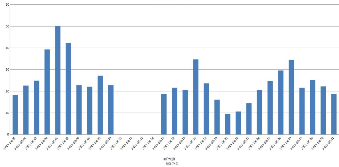
Старчево PM10
