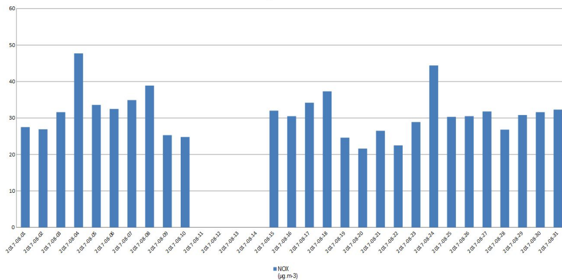
Старчево NOX
