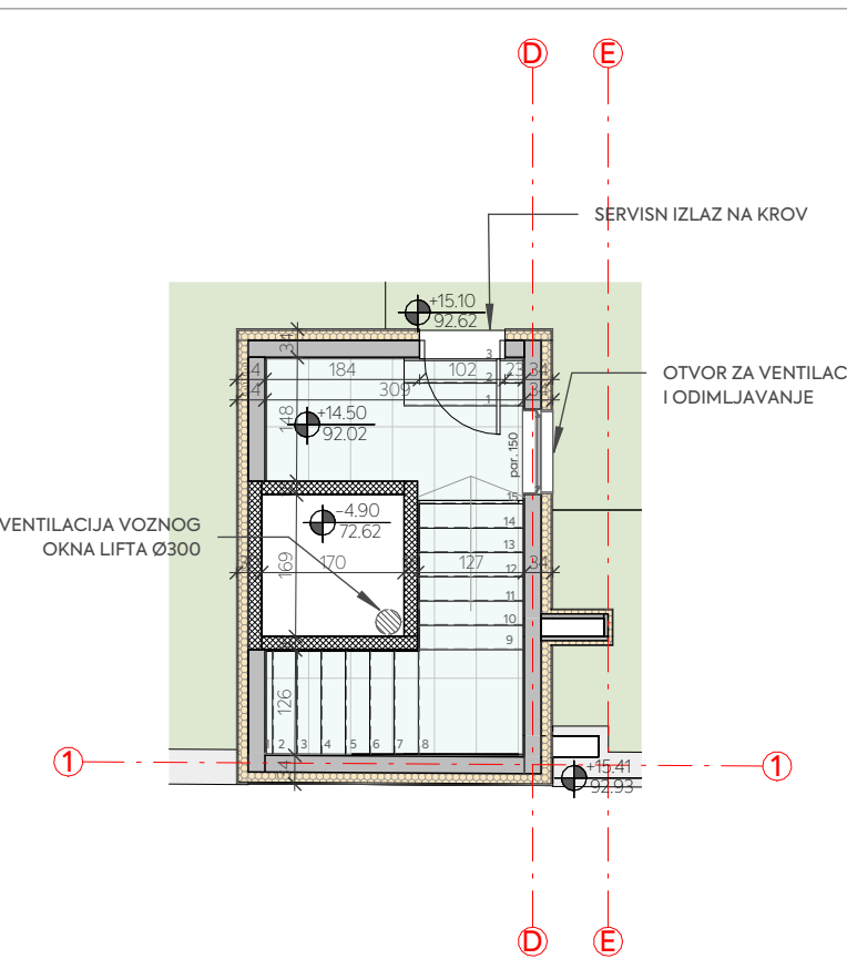
DETALJ SERVISNOG IZLAZA NA KROV LAMELE 1
