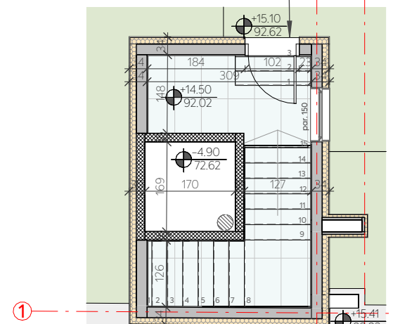
SERVISN IZLAZ NA KROV
