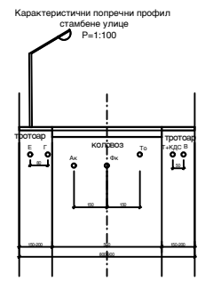
Карактеристични попречни профил стамбене улице R=1:100
