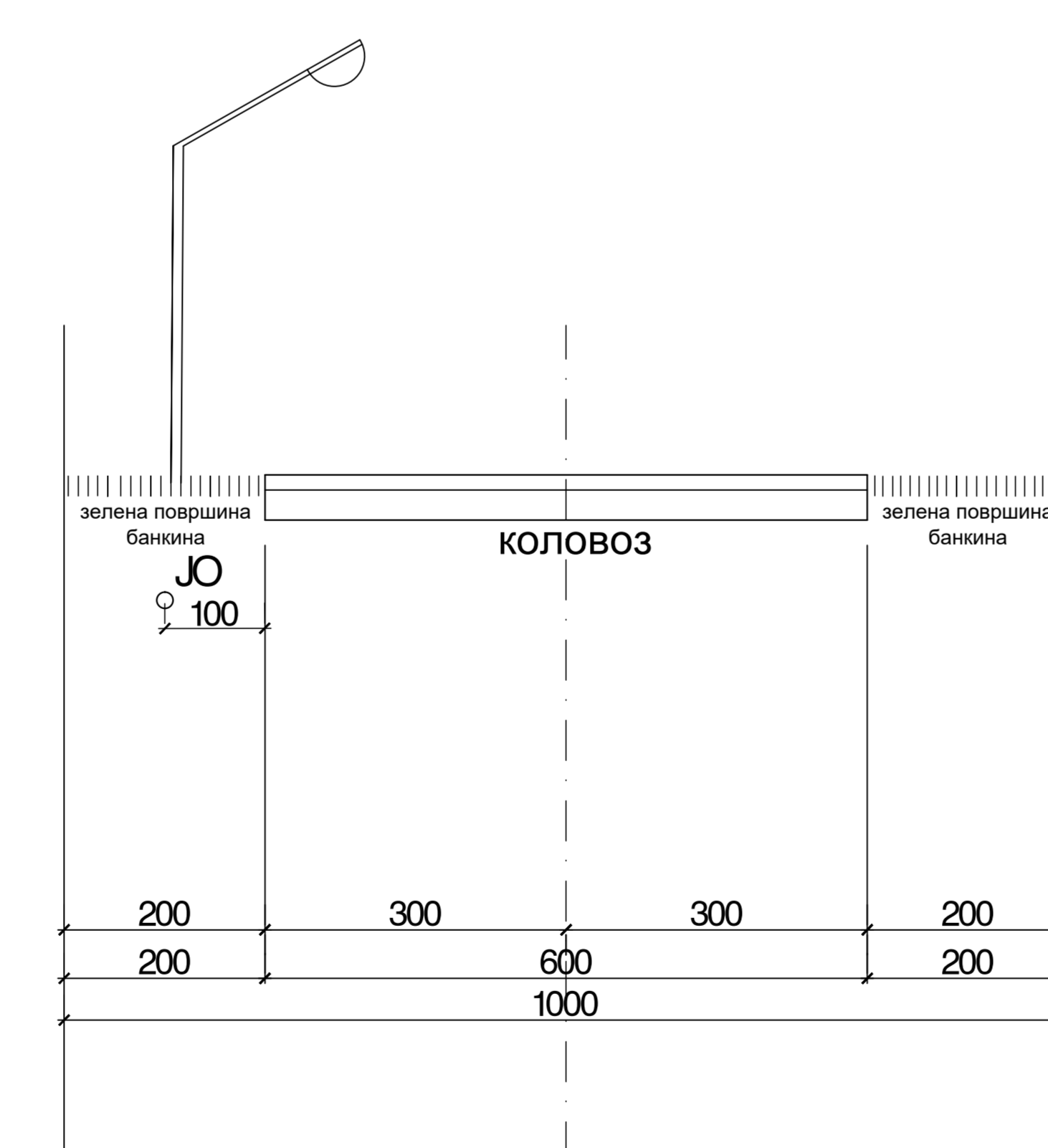
Попречни профил 3 - 3 Сервисна саобраћајница
