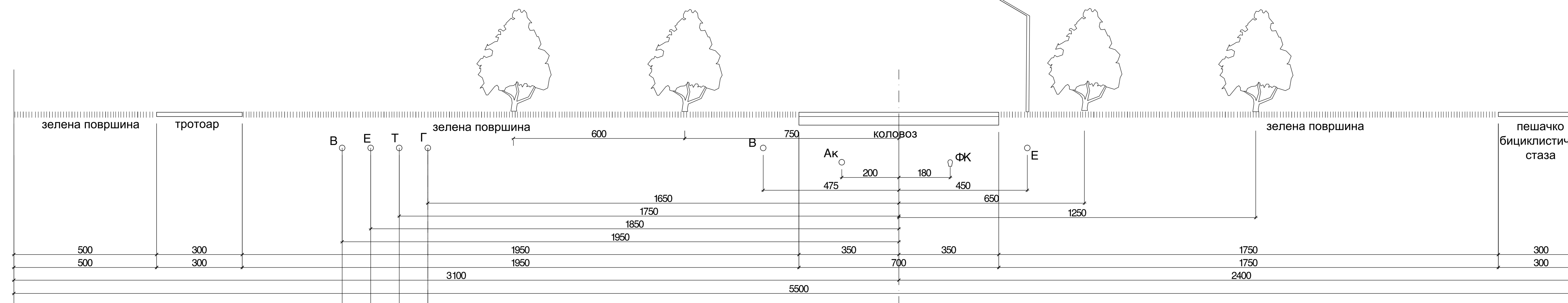
Попречни профил 1 - 1 Стари црепајски пут
