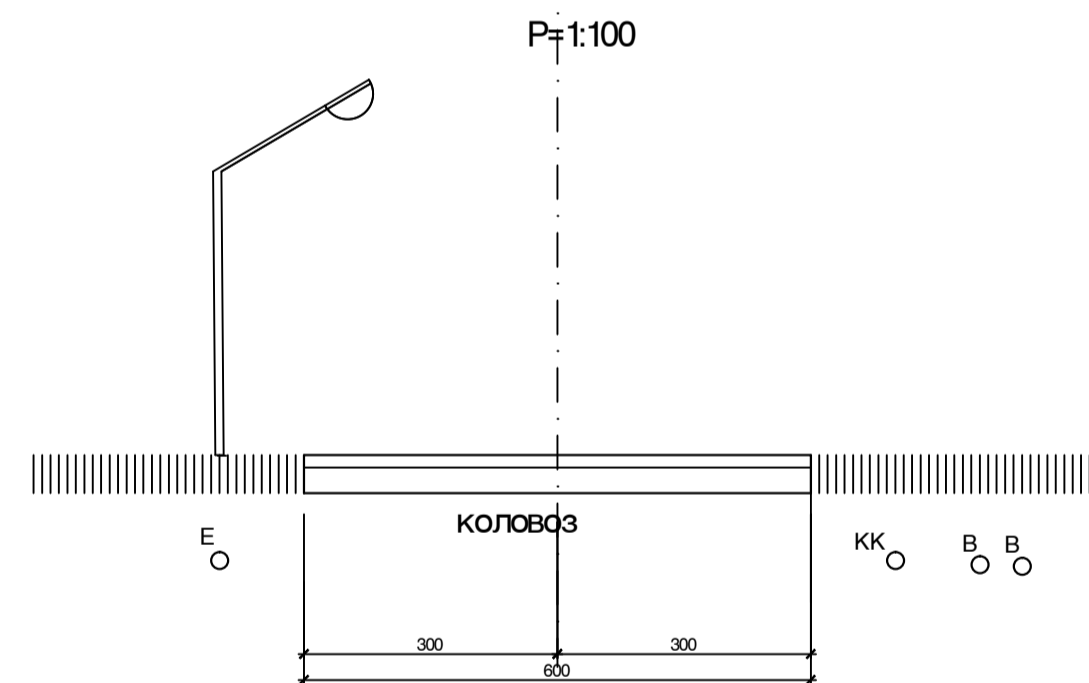
Карактеристични попречни профил 2 - 2
