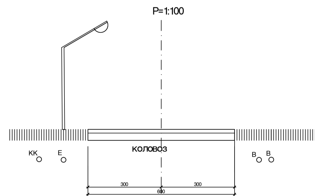
Карактеристични попречни профил 1 - 1
