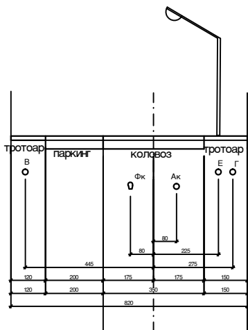
поперчни профил 2 - 2 P=1:100
