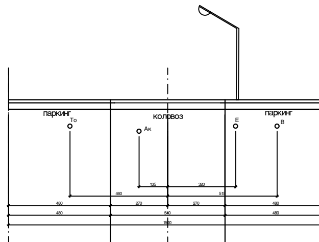
поперчни профил 4 - 4 P=1:100
