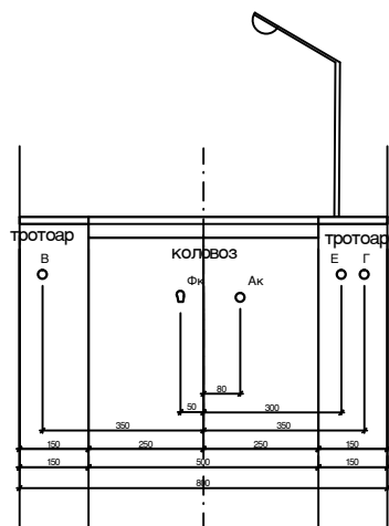
поперчни профил 1 - 1 P=1:100
