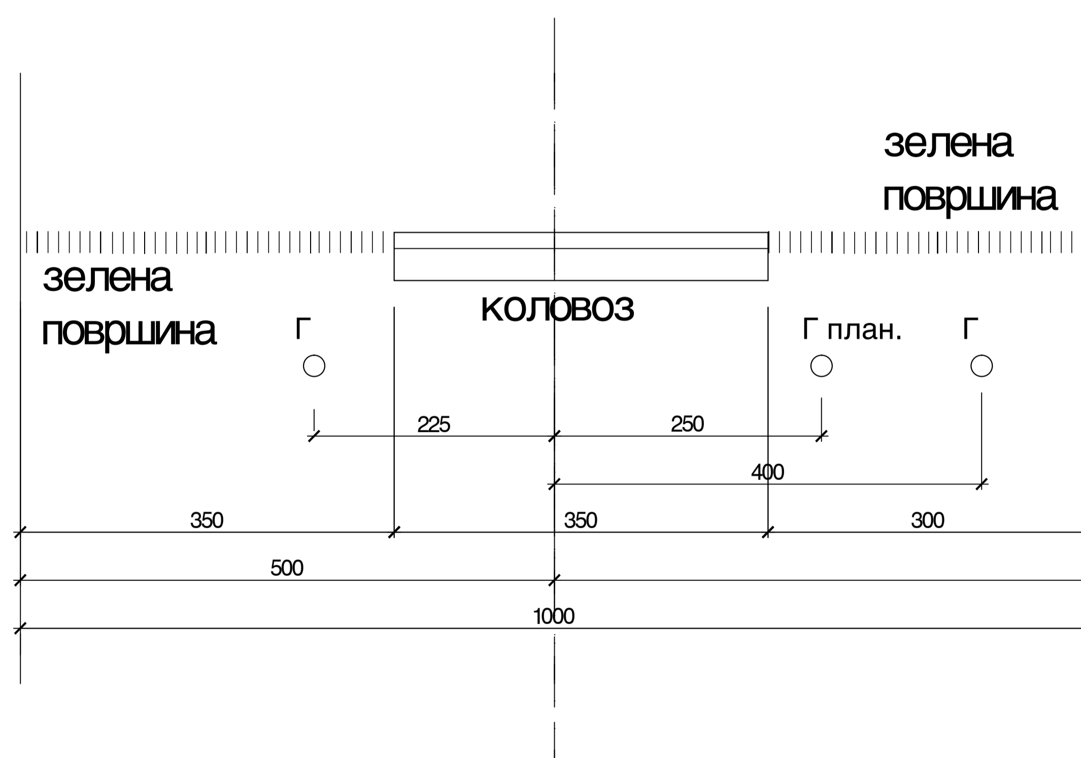
Карактеристични попречни профил 2 - 2 P=1:100
