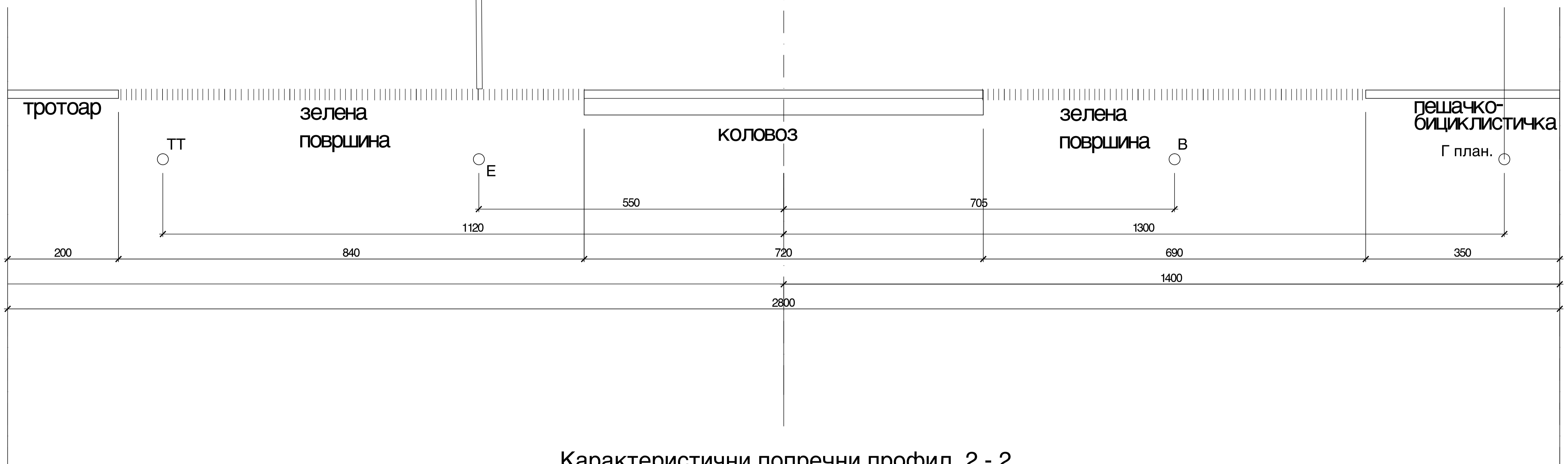
Карактеристични попречни профил 2 - 2 P=1:100
