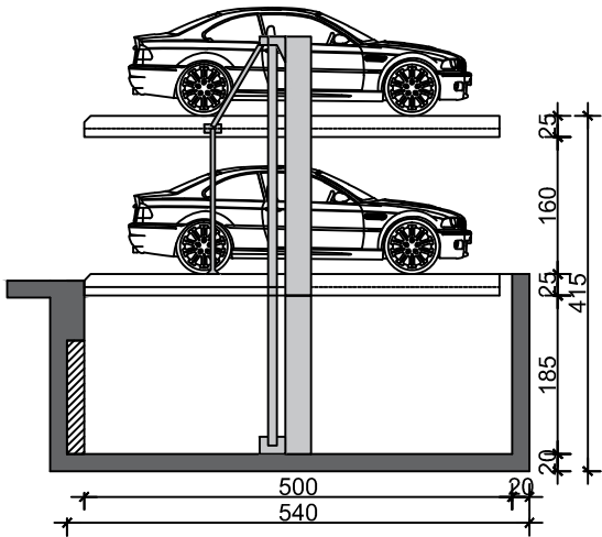
Presek 1-1
