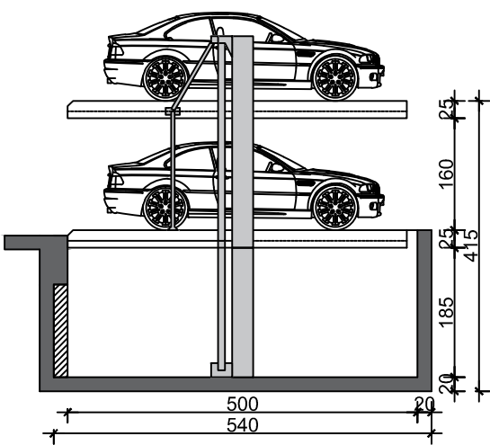
Presek 1-1
