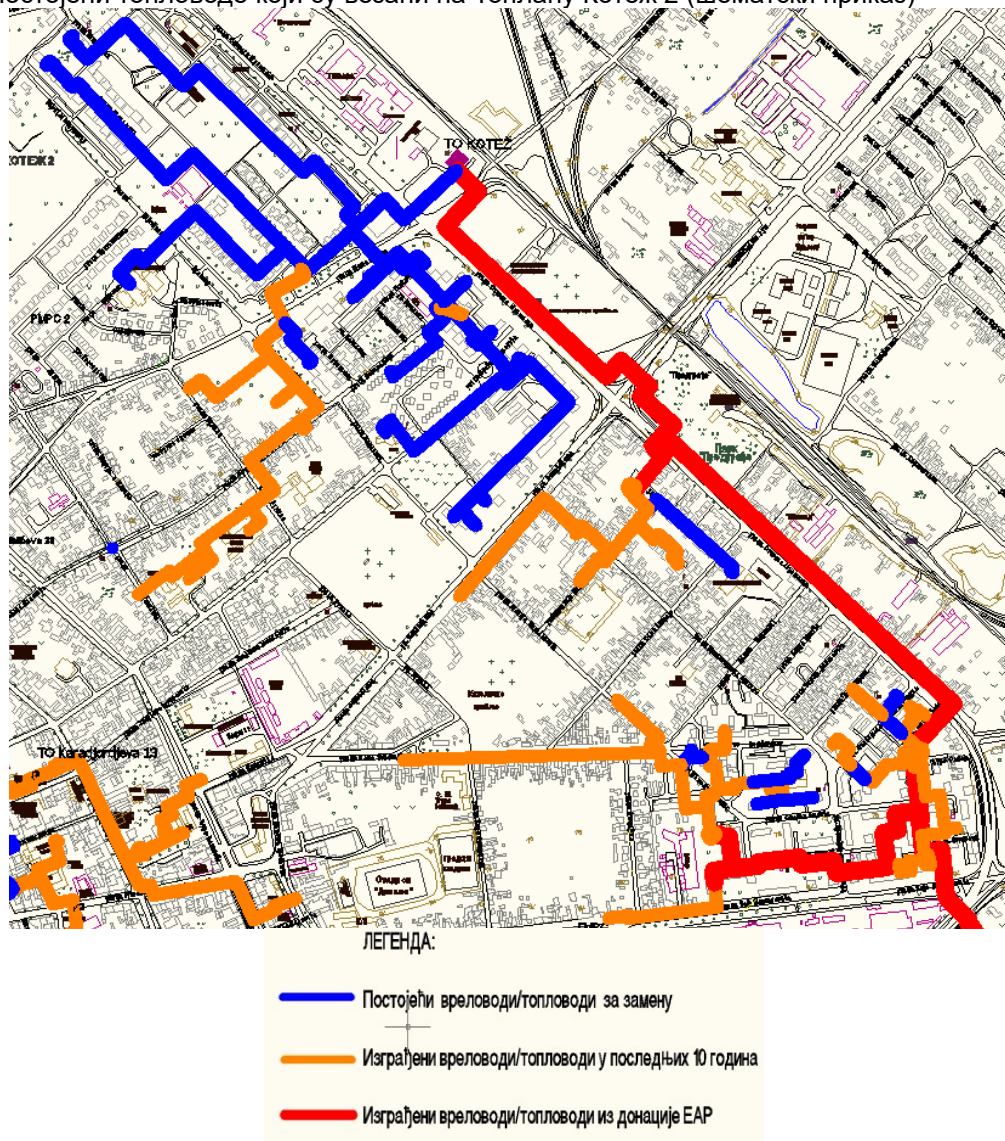
Слика 3. Постојећи топоводи који су везани на Топлану Котеж 2 (шематски приказ)
