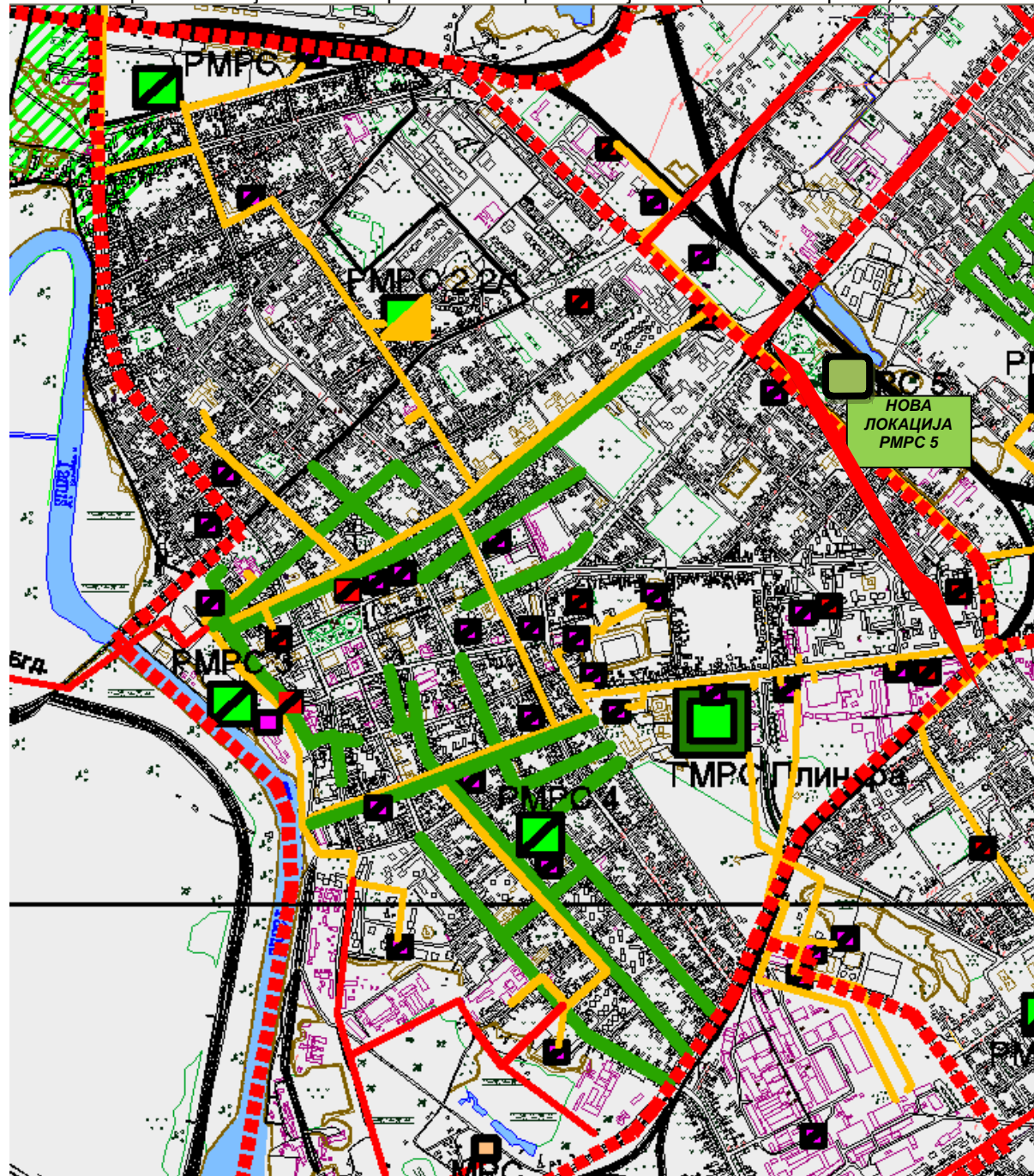
Слика 4. Приказ постојеће и планиране гасне мреже и објекта (шематски приказ)
