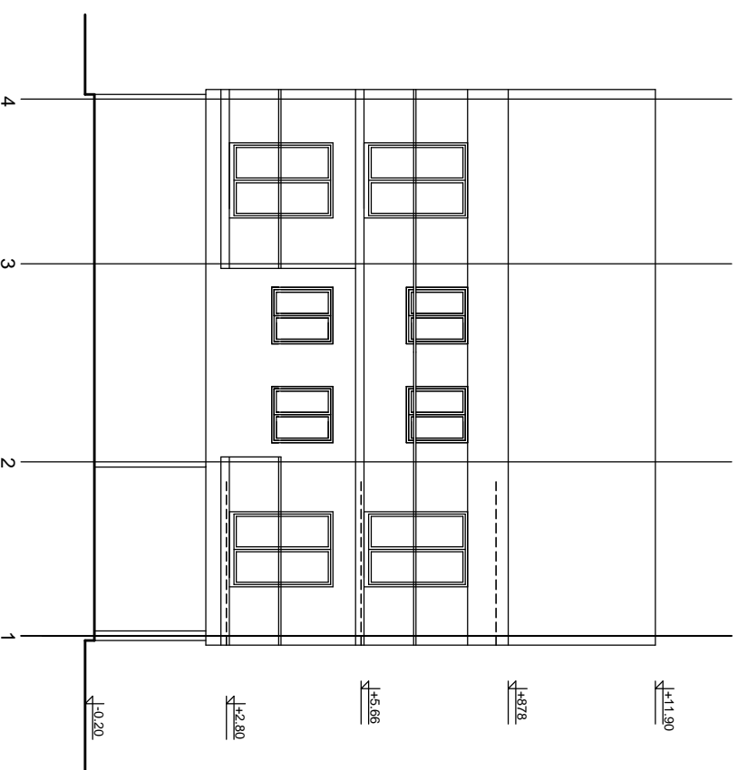
Jugoistocna fasada
