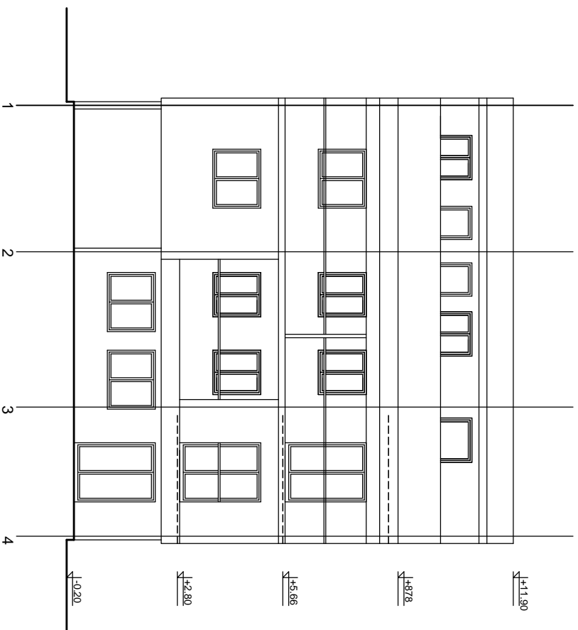
Severozapadna fasada
