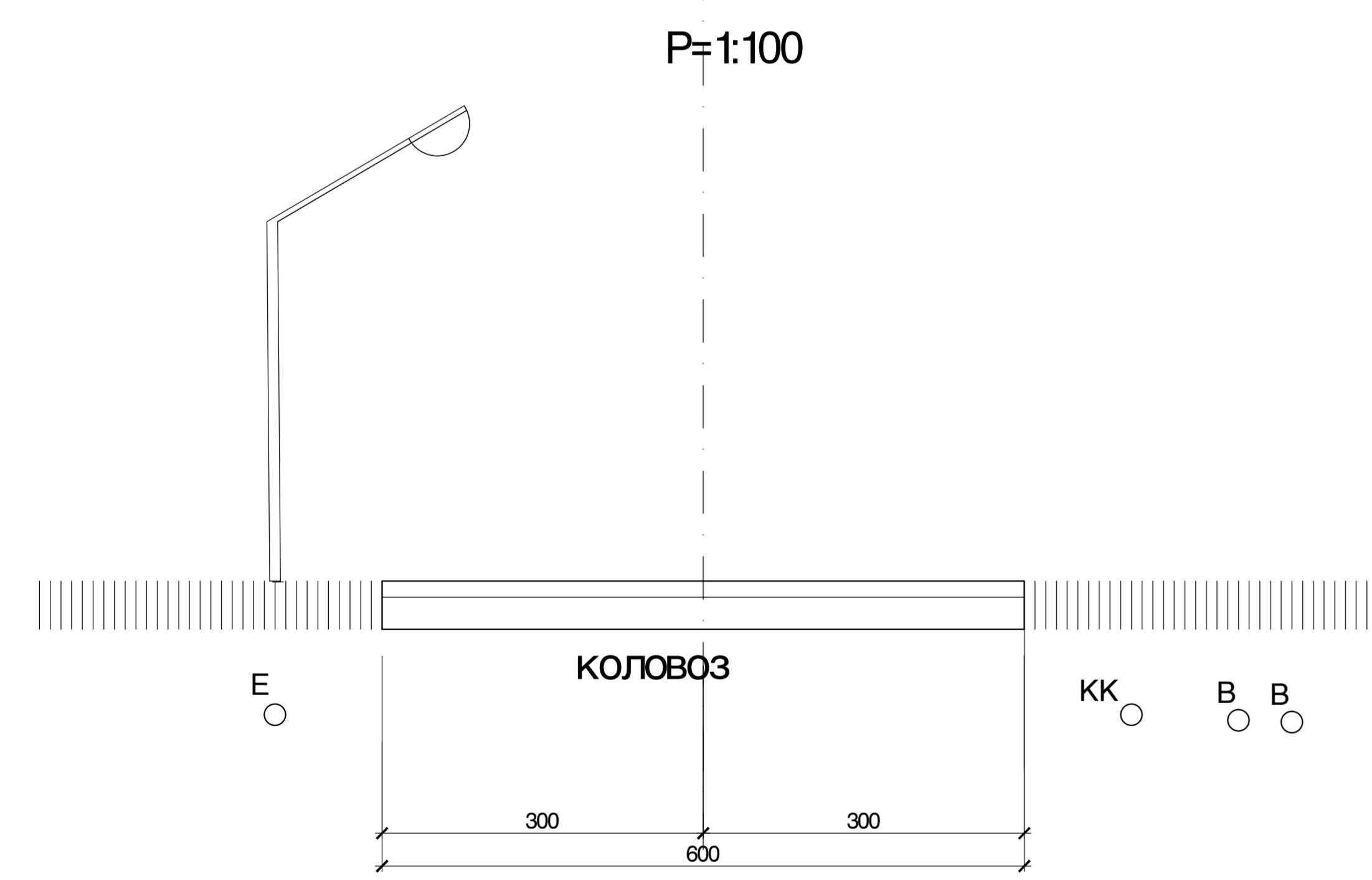
Карактеристични попрени профил 2 - 2
