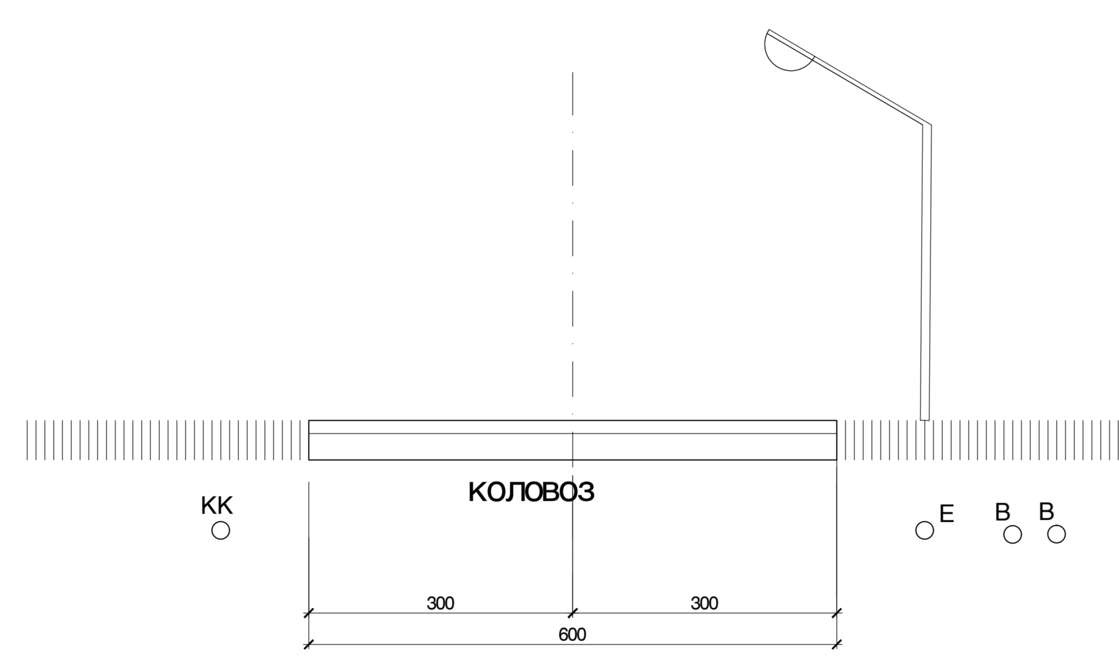
Карактеристични попрени профил 3 - 3
