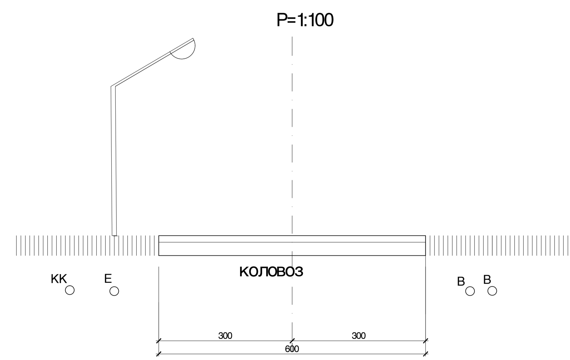
Карактеристични попрени профил 1 - 1
