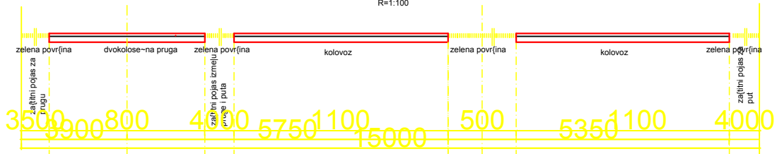
Poprečni profil 2-2 Drumsko - železni-ka obilaznica oko Panjeva R=1:100
