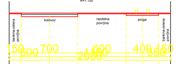
Poprečni profil 3-3 Drumsko - železni-ka saobraćajnica R=1:100
