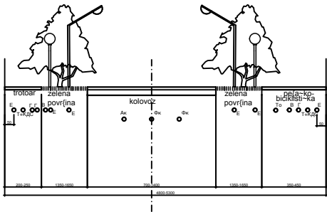
Karakteristični poprečni profil sa generalnim rasporedom infrastrukture glavne gradske ulice R=1:100
