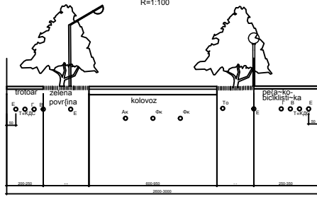
Karakteristični poprečni profil sa generalnim rasporedom infrastrukture Opštinskog puta R=1:100
