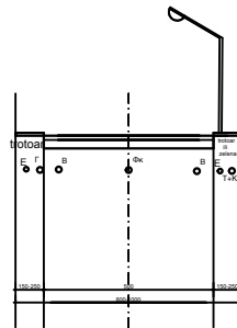
Karakteristični poprečni profil sa generalnim rasporedom infrastrukture kolosko - pešačka saobraćajnice R=1:100
