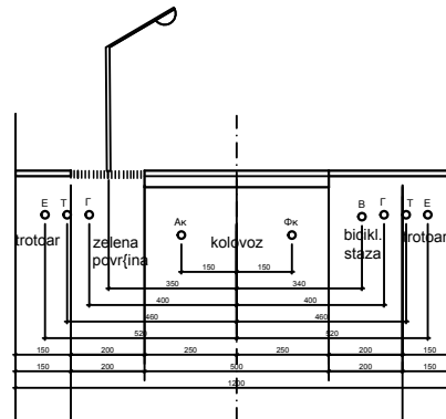
попечни профил сабирне улице 5 - 5 P=1:100
