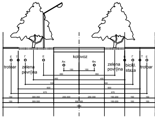
попечни профил сабирне улице 1 - 1 P=1:100
