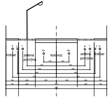
попечни профил стамбене улице 3 - 3 P=1:100
