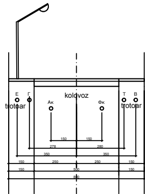
попечни профил стамбене улице 4 - 4 P=1:100
