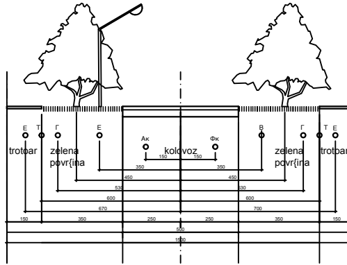
попечни профил стамбене улице 2 - 2 P=1:100
