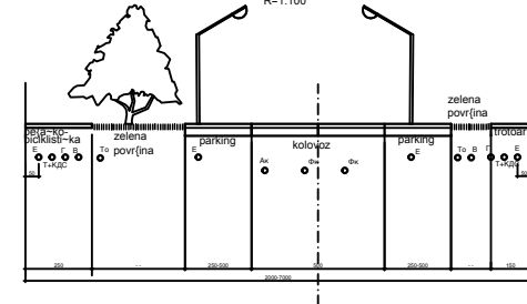
Karakteristični poprečni profil sa generalnim rasporedom infrastrukture stambene ulice R=1:100
