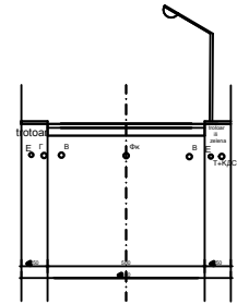
Karakteristični poprečni profil sa generalnim rasporedom infrastrukture integrisane saobraćajnice R=1:100
