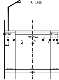
Karakteristični poprečni profil sa generalnim rasporedom infrastrukture stambene ulice R=1:100
