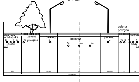
Karakteristični poprečni profil sa generalnim rasporedom infrastrukture sabirne ulice R=1:100
