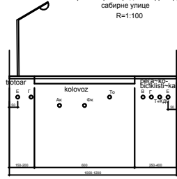
Karakteristični poprečni profil sa generalnim rasporedom infrastrukture sabirne ulice R=1:100
