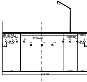
Karakteristični poprečni profil sa generalnim rasporedom infrastrukture sabirne ulice R=1:100
