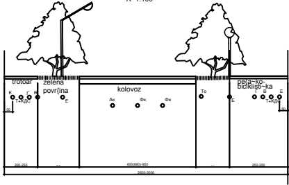
Karakteristični poprečni profil sa generalnim rasporedom infrastrukture Opštinskiog - lokalnog puta R=1:100
