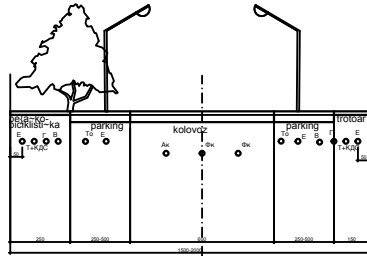
Karakteristični poprečni profil sa generalnim rasporedom infrastrukture sabirne ulice R=1:100
