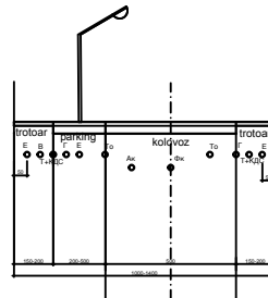
Karakteristični poprečni profil sa generalnim rasporedom infrastrukture stambene ulice R=1:100
