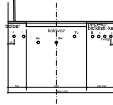
Karakteristični poprečni profil sa generalnim rasporedom infrastrukture stambene ulice R=1:100
