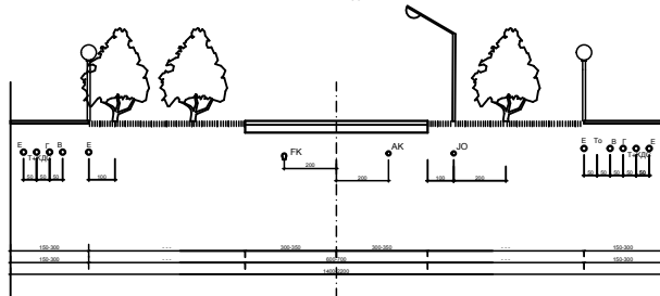
Karakteristični poprečni profil zonskih saobraćajnica R=1:100
