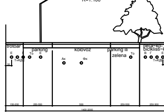
Karakteristični poprečni profil sa generalnim rasporedom infrastrukture stambene ulice R=1:100
