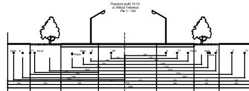
Поперечный профиль 13-13 д. Милош. Телькина Ры 1:100
