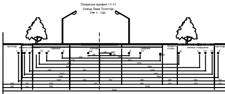
Поперечный профиль 11-11 Улицы Давы. Толстого Ры 1:100
