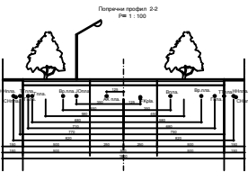
Поперечный профиль 2-2 Ры 1:100
