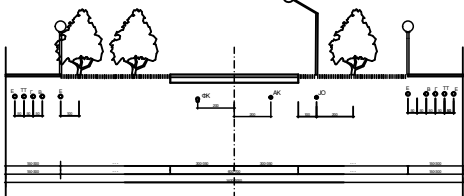
Карактеристични попречни профил зонских саобраћајница R=1:100
