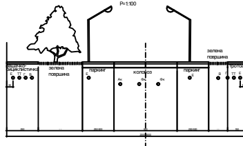
Карактеристични попречни профил са генералним распоредом инфраструктуре стабилне улице R=1:100
