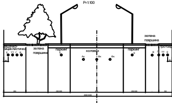
Карактеристични попречни профил са генералним распоредом инфраструктуре сабирне улице R=1:100
