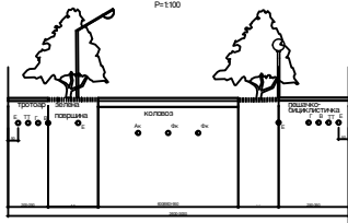
Карактеристични попречни профил са генералним распоредом инфраструктуре Општински - локални путева R=1:100
