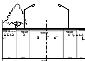
Карактеристични попречни профил са генералним распоредом инфраструктуре сабирне улице R=1:100
