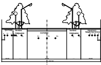
Карактеристични попречни профил са генералним распоредом инфраструктуре главних наредних улица R=1:100
