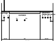
Карактеристични попречни профил са генералним распоредом инфраструктуре сабирне улице R=1:100
