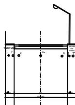
Карактеристични попречни профил са генералним распоредом инфраструктуре копно - пешачке саобраћајнице R=1:100
