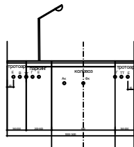
Карактеристични попречни профил са генералним распоредом инфраструктуре стабилне улице R=1:100
