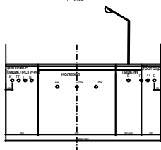
Карактеристични попречни профил са генералним распоредом инфраструктуре сабирне улице R=1:100
