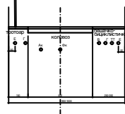
Карактеристични попречни профил са генералним распоредом инфраструктуре стабилне улице R=1:100
