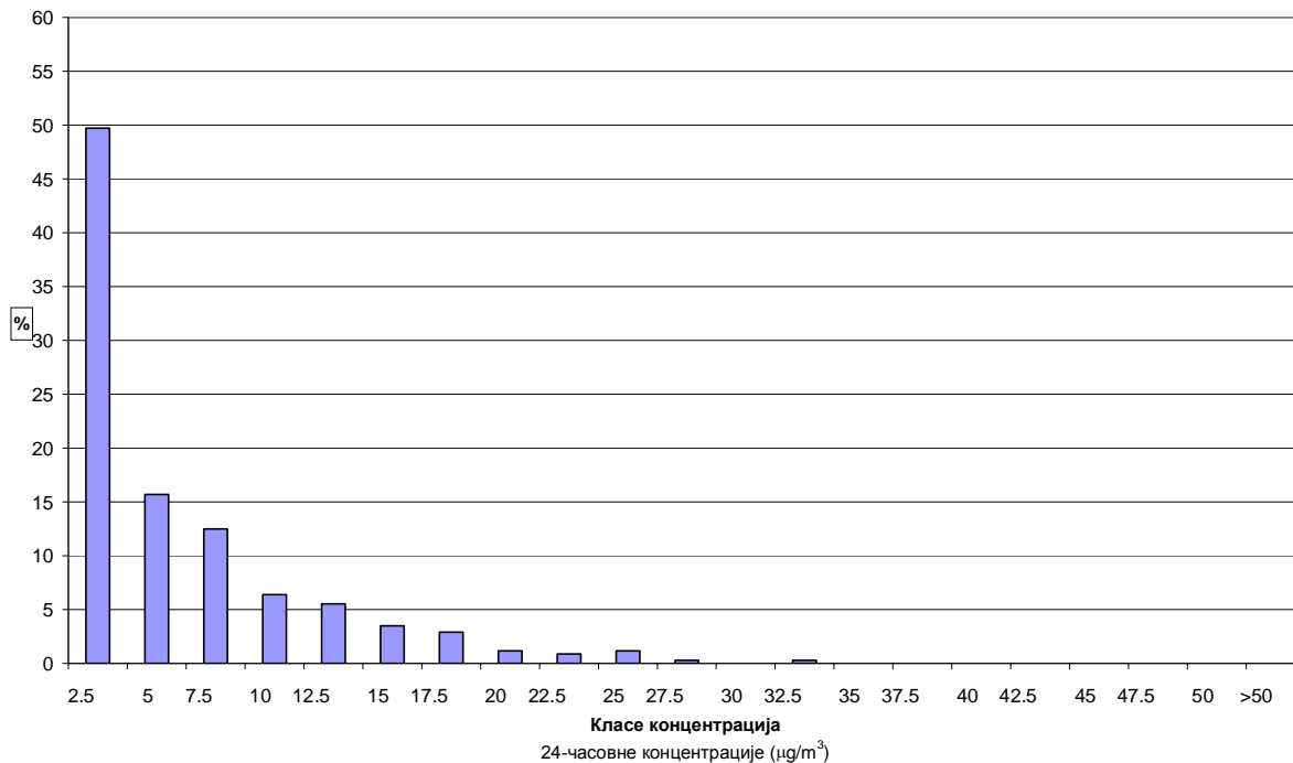
Чађ у ваздуху амбијента Мерно место, Панчево-Стрелиште 2015. год. Дистрибуција релативних фреквенција UV појединачно у ваздуху
