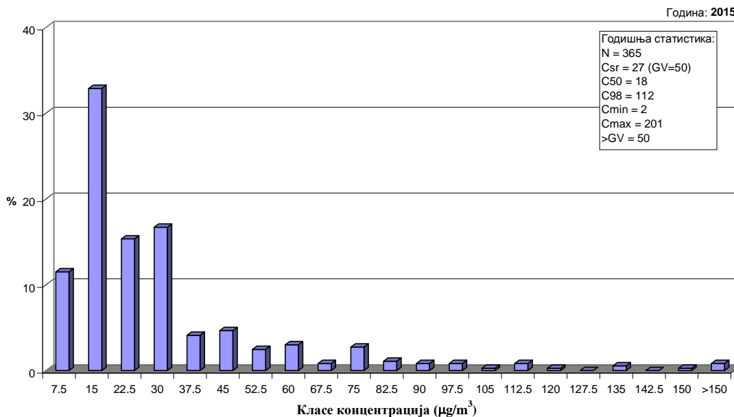
Чај у ваздуху амбијента Мерно место Стрелиште, Панчево Дистрибуција релативних фреквенција 24h концентрација
