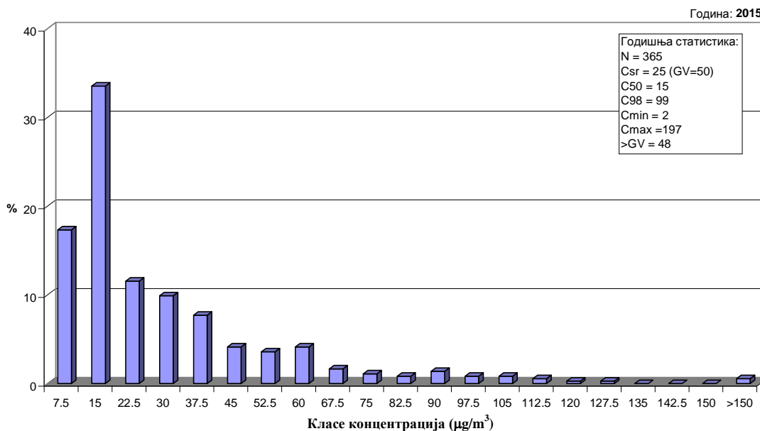
Чај у ваздуху амбијента Мерно место Нова Миса, Панчево Дистрибуција релативних фреквенција 24h концентрација
