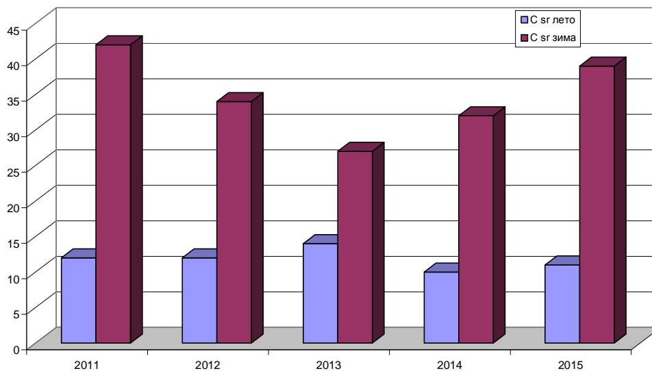
Чађ у ваздуху амбијента мерно место Стрелиште, Панчево Упоредни вишегодишњи приказ просечних сезонских концентрација у \mu\text{g}/\text{m}^3
