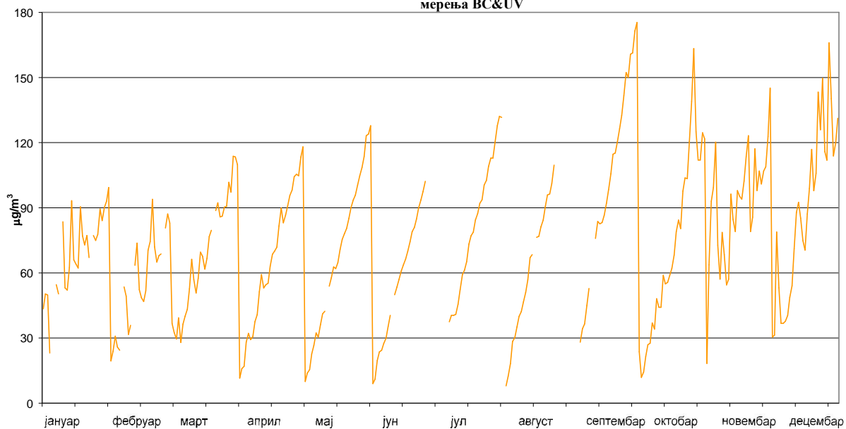
ЧАБ у ваздуху амбијента Мерно место Стрелиште, 2015. година Приказ 24h концентрација прерачуната корелацијом на основу резултата континуалних мерења BC&UV
