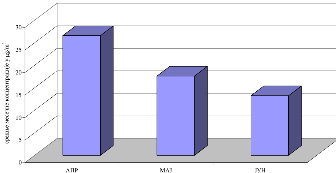
PM 2.5 у ваздуху амбијента Мерно место: Панчево, Народна башта II квартал 2016.године Сезонска дистрибуција средњих месечних концентрација (µg/m 3 ) аутоматски мониторинг
