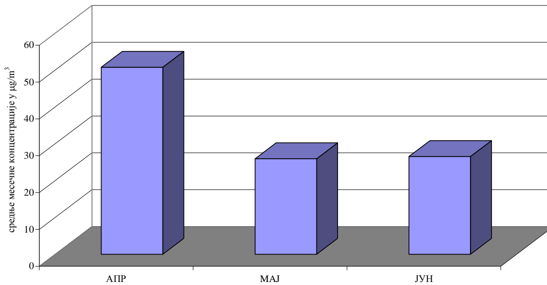
PM 10 у ваздуху амбијента Мерино место: Панчево, Народна башта II квартал 2016.године Сезонска дистрибуција средњих месечних концентрација (µg/m³) аутоматски мониторинг
