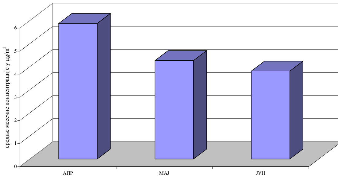
Ксилен у ваздуху амбијента Мерно место: Панчево, Народна башта II квартал 2016.године Сезонска дистрибуција средњих месечних концентрација ( \mu\text{g}/\text{m}^3 ) аутоматски мониторинг
