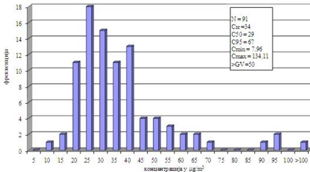
PM 10 у ваздуху амбијента Мерно место: Панчево, Народна башта II квартал 2016. године Дистрибуција релативних фреквенција 24h концентрација аутоматски мониторинг
