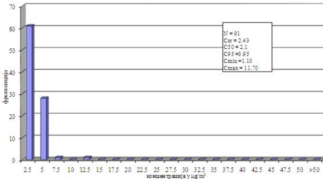
Толуен у ваздуху амбијента Мерно место: Панчево, Народна башта II квартал 2016. године Дистрибуција релативних фреквенција 24h концентрација аутоматски мониторинг
