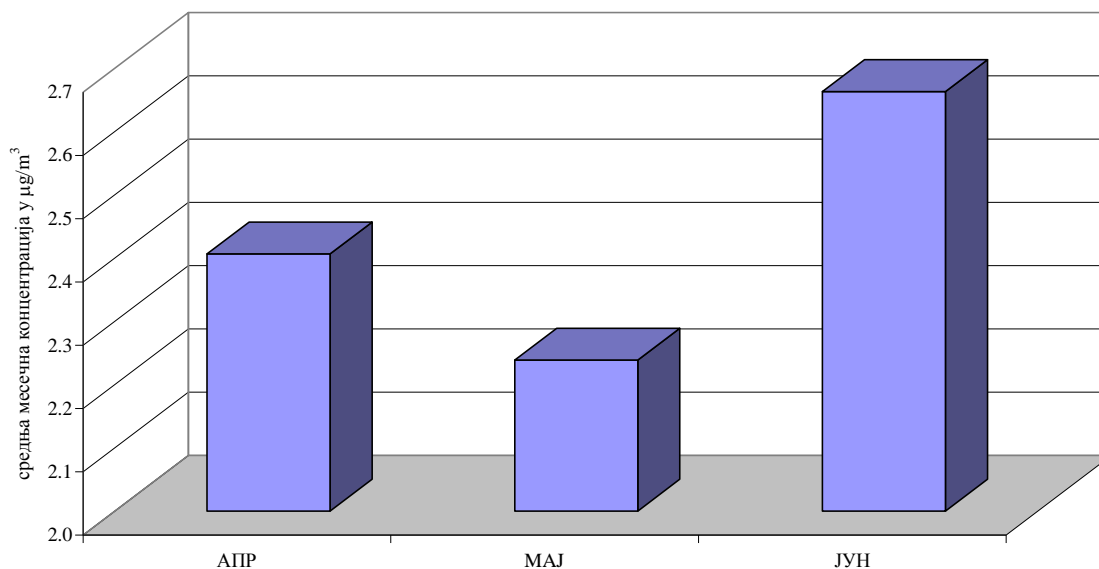
Толуен у ваздуху амбијента Мерно место: Панчево, Народна башта II квартал 2016.године Сезонска дистрибуција средњих месечних концентрација ( \mu\text{g}/\text{m}^3 ) аутоматски мониторинг
