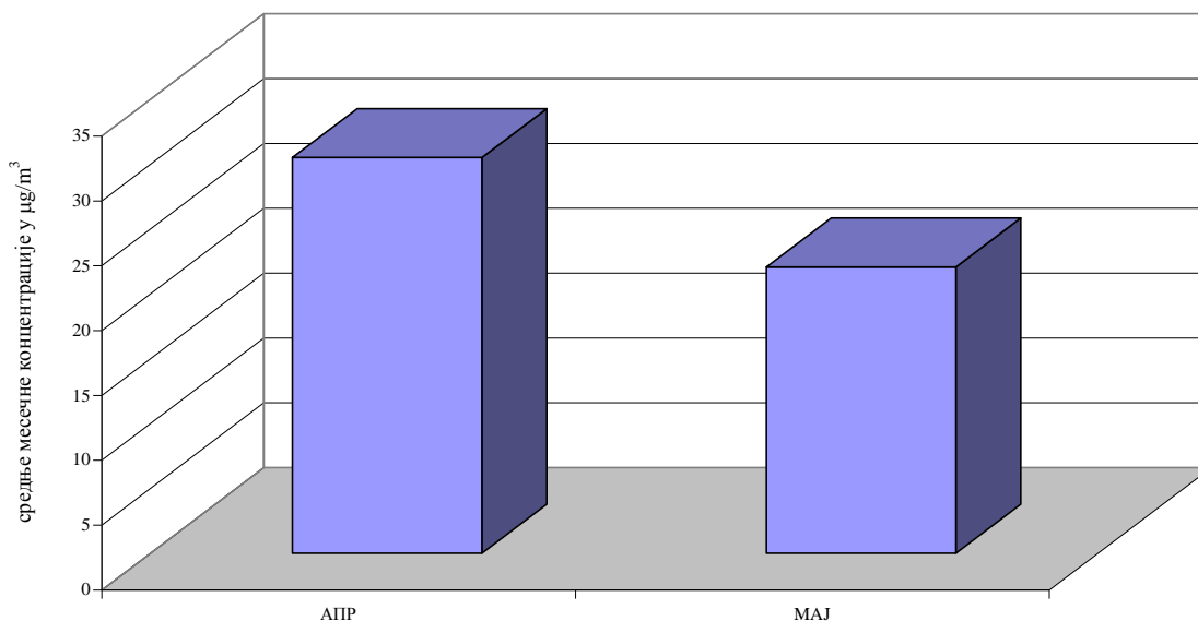
Азотни оксиди у ваздуху амбијента Мерно место: Панчево, Народна башта II квартал 2016.године Сезонска дистрибуција средњих месечних концентрација ( \mu\text{g}/\text{m}^3 ) аутоматски мониторинг
