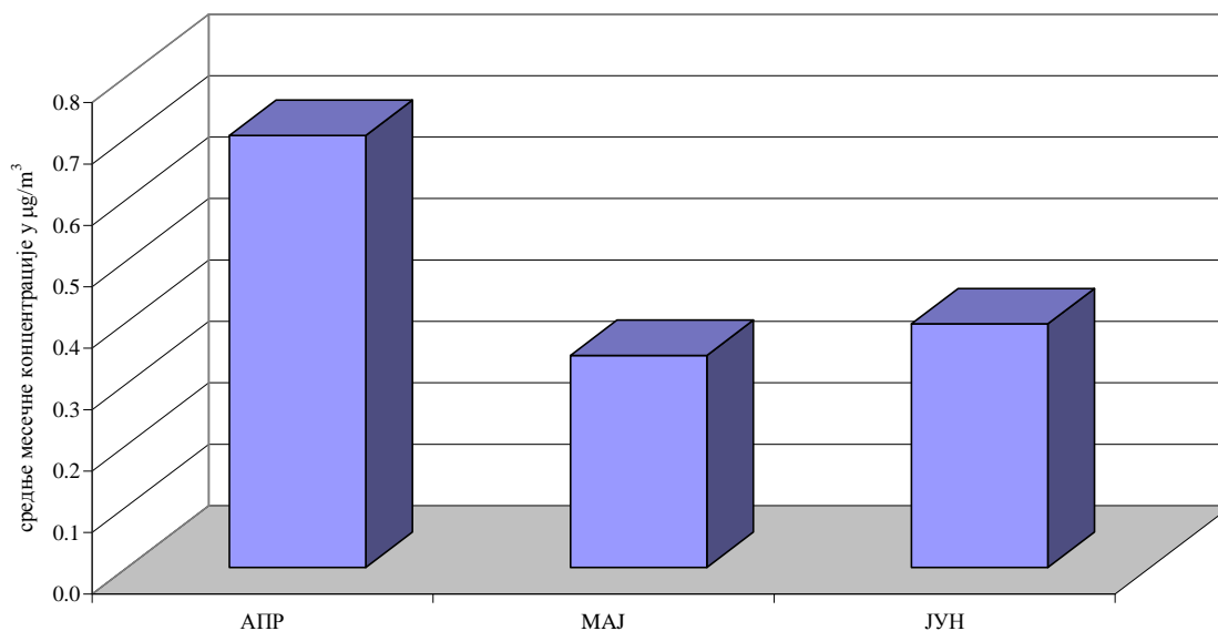
Бензен у ваздуху амбијента Мерно место: Панчево, Народна башта II квартал 2016.године Сезонска дистрибуција средњих месечних концентрација ( \mu\text{g}/\text{m}^3 ) аутоматски мониторинг
