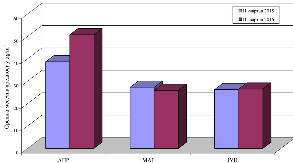
PM 10 У ВАЗДУХУ АМБИЈЕНТА Мерно место: Панчево, Народна башта Упоредни приказ просечних месечних концентрација у \mu\text{g}/\text{m}^3 II квартал 2015. - II квартал 2016.
