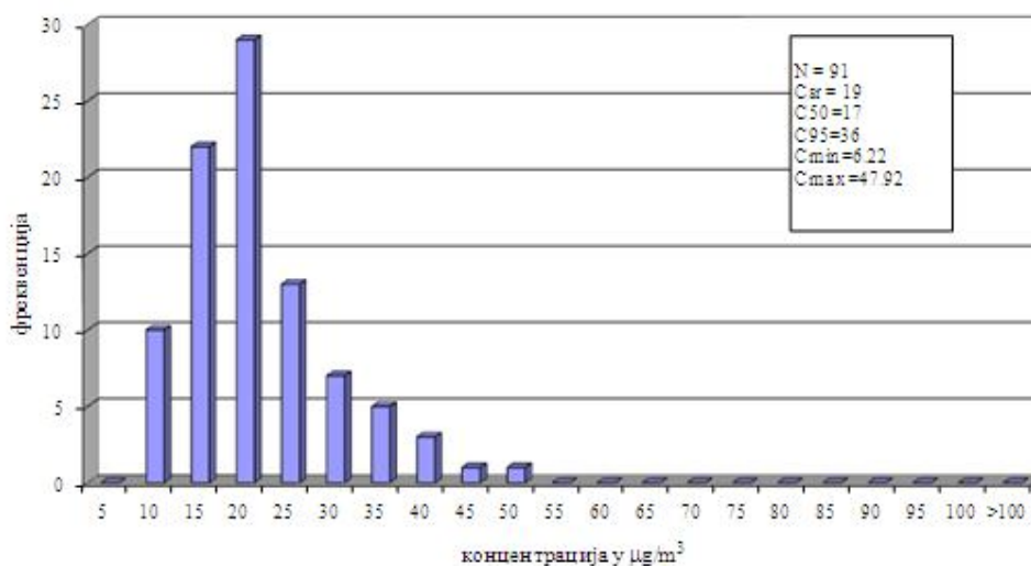
PM 2.5 у ваздуху амбијента Мерно место: Панчево, Народна башта II квартал 2016. године Дистрибуција релативних фреквенција 24h концентрација аутоматски мониторинг
