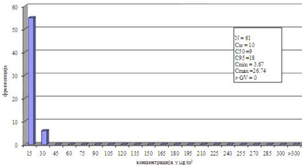
NH 3 у ваздуху амбијента Мерино место: Панчево, Народна башта II квартал 2016.године Дистрибуција релативних фреквенција 24h концентрација аутоматски мониторинг
