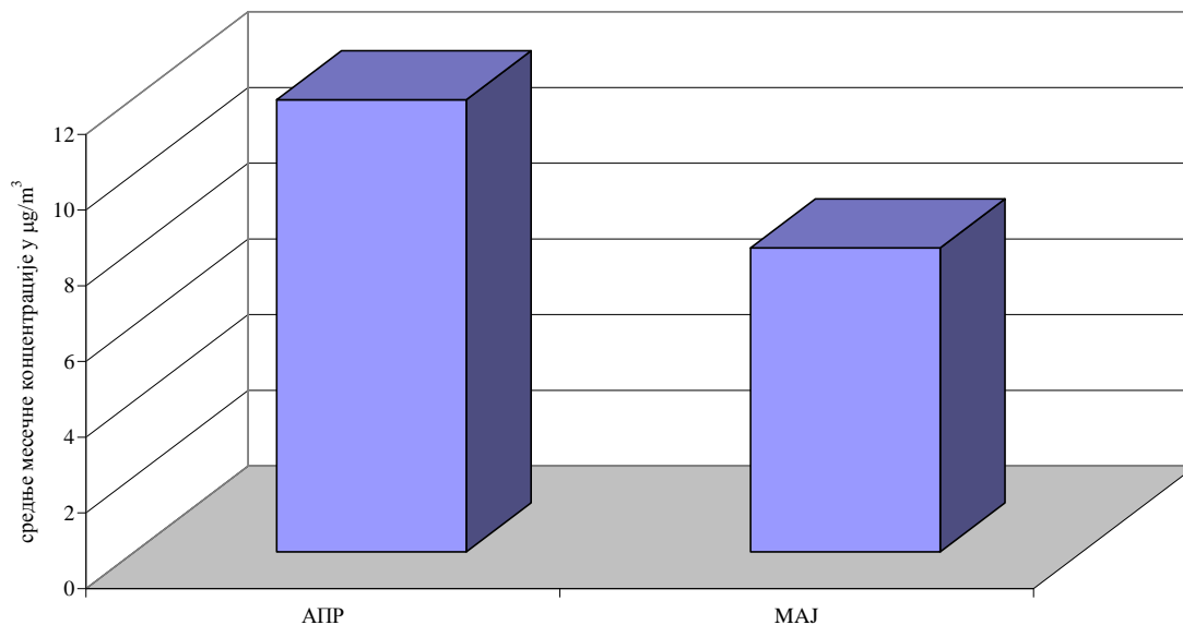
Амонијак у ваздуху амбијента Мерно место: Панчево, Народна башта II квартал 2016.године Сезонска дистрибуција средњих месечних концентрација (µg/m 3 ) аутоматски мониторинг
