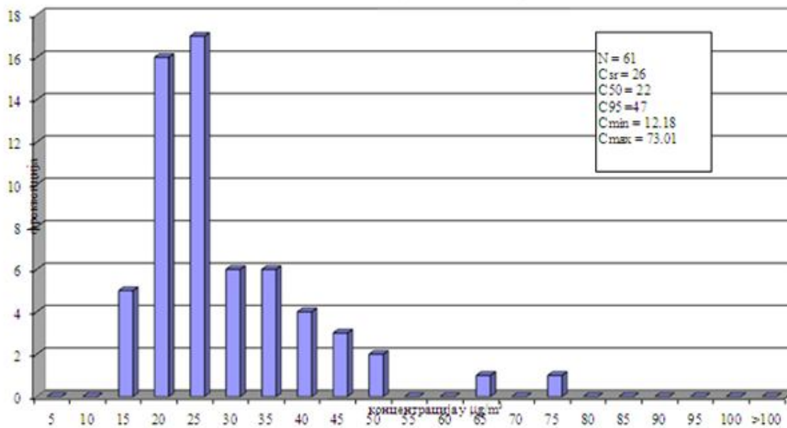
NOx у ваздуху амбијента Мерино место: Панчево, Народна башта II квартал 2016.године Дистрибуција релативних фреквенција 24h концентрација аутоматски мониторинг
