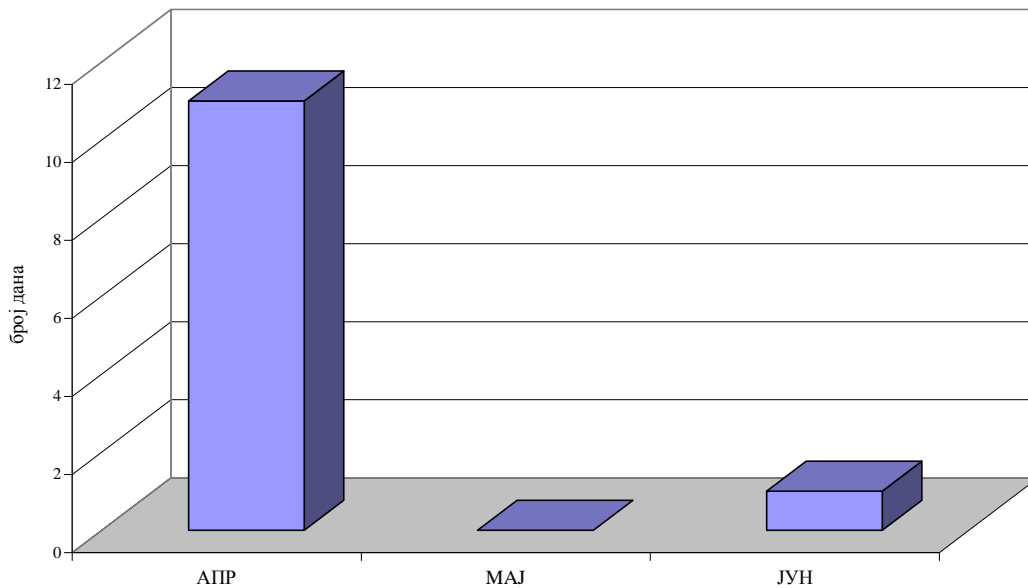
PM 10 У ВАЗДУХУ АМБИЈЕНТА Мерно место: Панчево, Народна башта Број дана са концентрацијама PM 10 изнад GV II квартал 2016.
