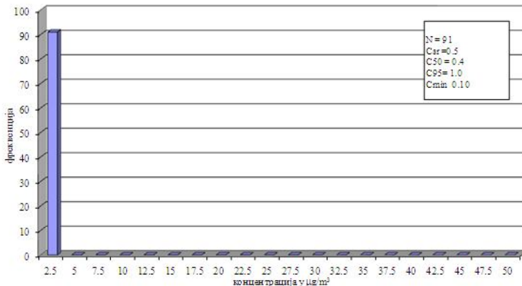
Бензен у ваздуху амбијента Мерно место: Панчево-Народна башта II квартал 2016. године Дистрибуција релативних фреквенција 24h концентрација аутоматски мониторинг
