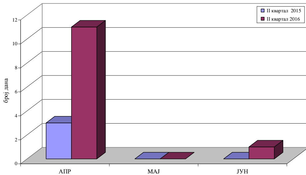
PM 10 У ВАЗДУХУ АМБИЈЕНТА Мерно место: Панчево, Народна башта Упоредни приказ броја дана са концентрацијама изнад GV II квартал 2015.-II квартал 2016.
