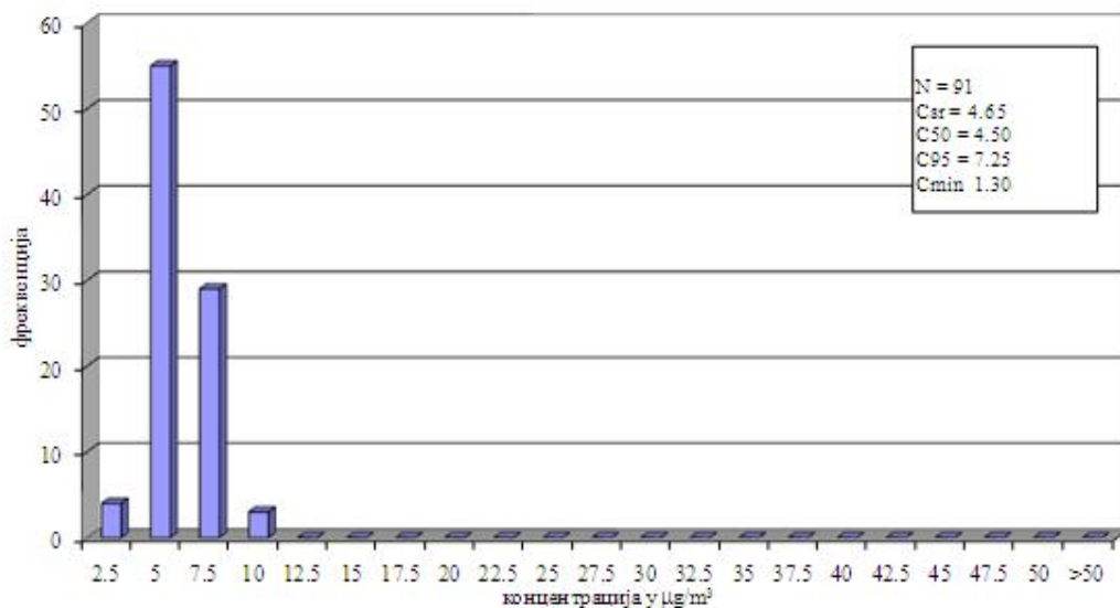
Кислород у ваздуху амбијента Мерино место :Панчево, Народна башта II квартал 2016.године Дистрибуција релативних фреквенција 24h концентрација аутоматски мониторинг
