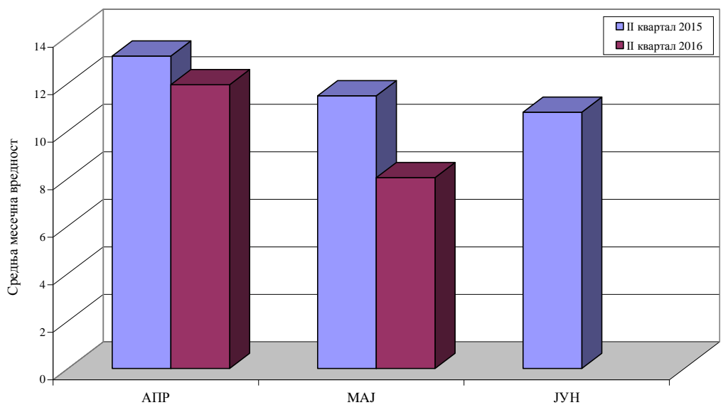
АМОНИЈАК У ВАЗДУХУ АМБИЈЕНТА Мерно место: Панчево, Народна башта Упоредни приказ просечних месечних концентрација у \mu\text{g}/\text{m}^3 II квартал 2015. - II квартал 2016.
