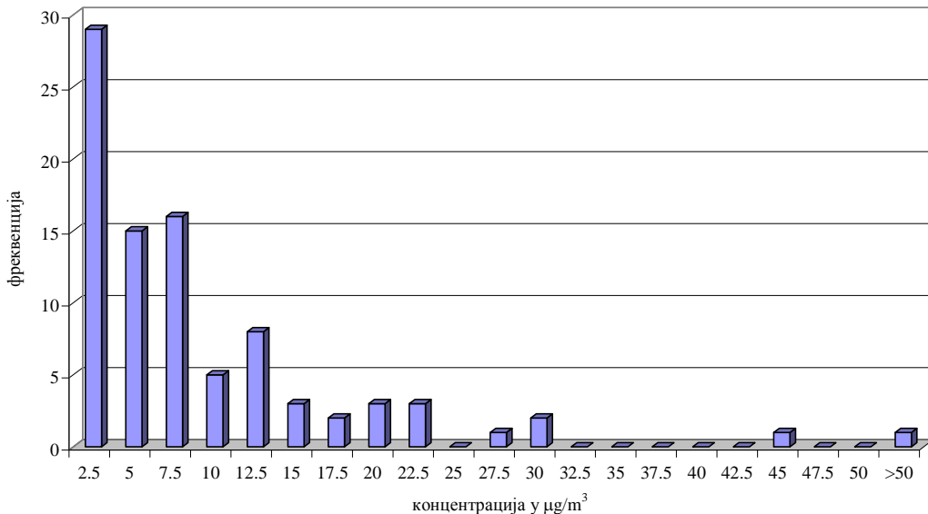
Толуен у ваздуху амбијента Мерно место :Панчево, Народна башта I квартал 2016.године Дистрибуција релативних фреквенција 24h концентрација аутоматски мониторинг
