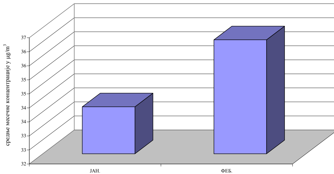
Азотни оксиди у ваздуху амбијента Мерно место: Панчево, Народна башта I квартал 2016.године Сезонска дистрибуција средњих месечних концентрација ( \mu\text{g}/\text{m}^3 ) аутоматски мониторинг
