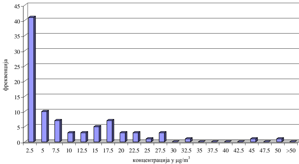
Ксилен у ваздуху амбијента Мерно место :Панчево, Народна башта I квартал 2016.године Дистрибуција релативних фреквенција 24h концентрација аутоматски мониторинг
