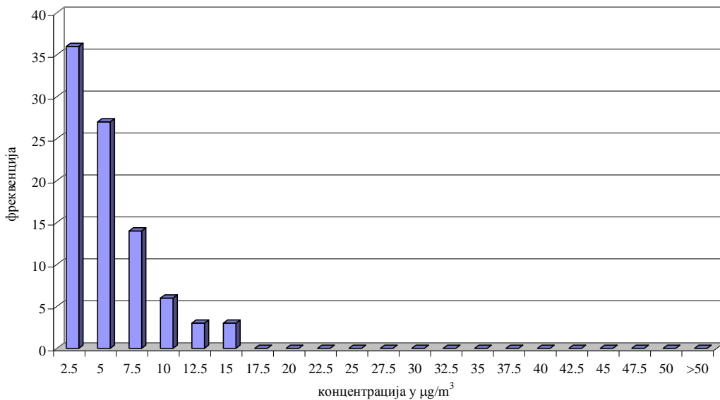
Бензен у ваздуху амбијента Мерно место: Панчево-Народна башта I квартал 2016. године Дистрибуција релативних фреквенција 24h концентрација аутоматски мониторинг
