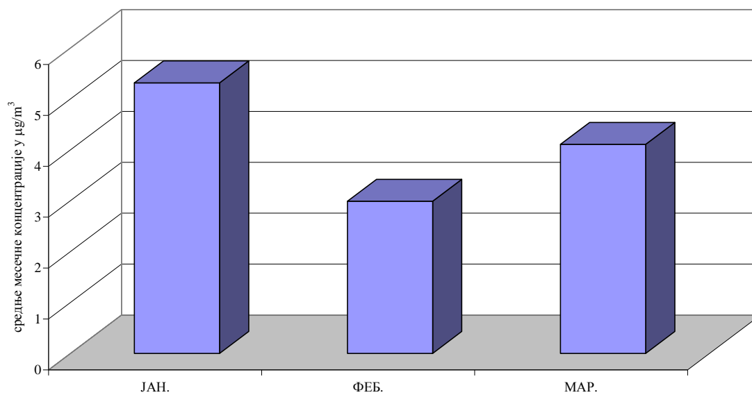
Бензен у ваздуху амбијента Мерно место: Панчево, Народна башта I квартал 2016.године Сезонска дистрибуција средњих месечних концентрација ( \mu\text{g}/\text{m}^3 ) аутоматски мониторинг
