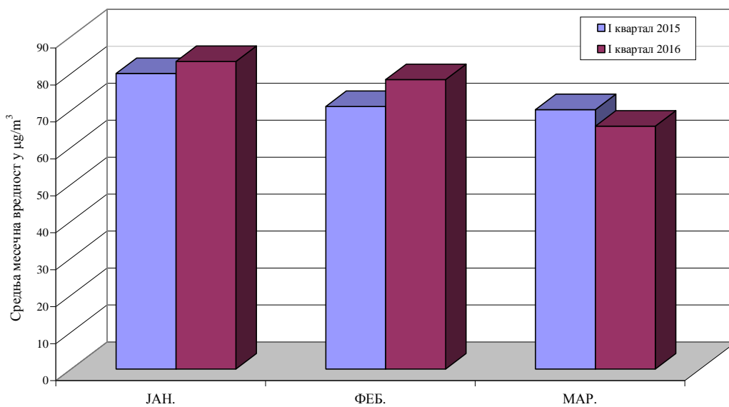
PM10 У ВАЗДУХУ АМБИЈЕНТА Мерно место: Панчево, Народна башта Упоредни приказ просечних месечних концентрација у \mu\text{g}/\text{m}^3 I квартал 2015. - I квартал 2016.
