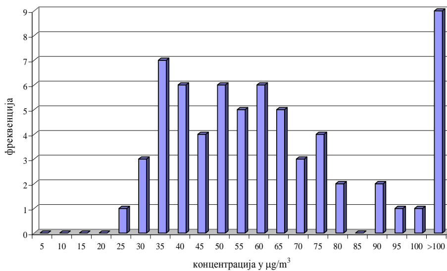
PM2,5 у ваздуху амбијента Мерно место: Панчево, Народна башта I квартал 2016.године Дистрибуција релативних фреквенција 24h концентрација аутоматски мониторинг
