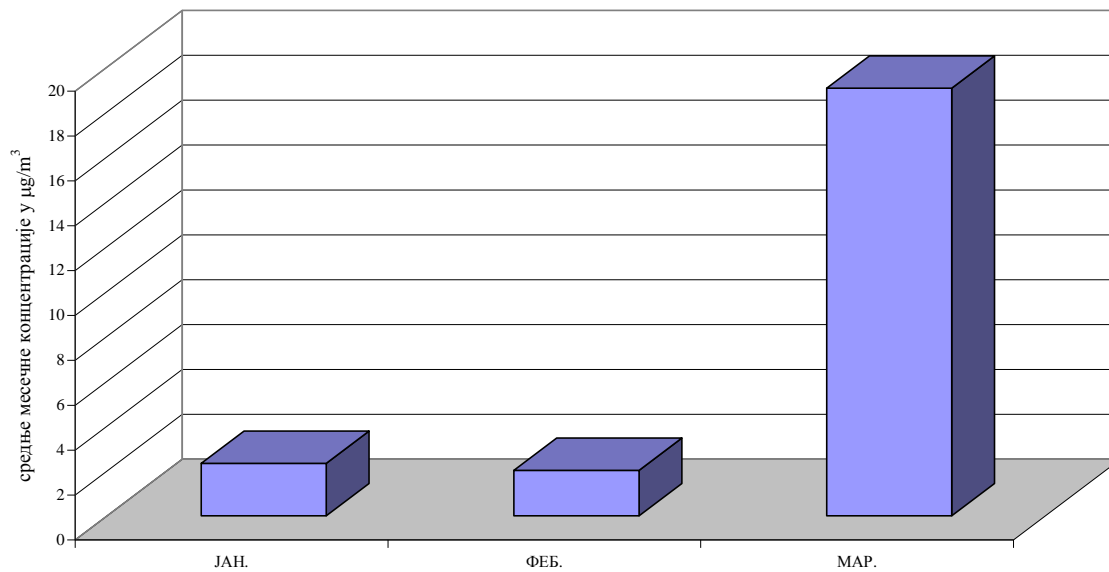
Ксилен у ваздуху амбијента Мерно место: Панчево, Народна башта I квартал 2016.године Сезонска дистрибуција средњих месечних концентрација ( \mu\text{g}/\text{m}^3 ) аутоматски мониторинг
