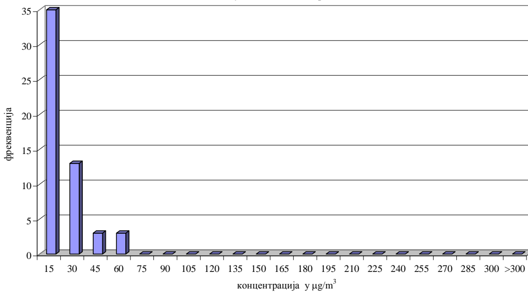
NO 2 у ваздуху амбијента Мерно место: Панчево, Народна башта I квартал 2016.године Дистрибуција релативних фреквенција 24h концентрација аутоматски мониторинг
