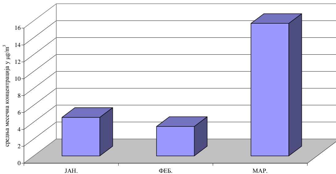
Толуен у ваздуху амбијента Мерно место: Панчево, Народна башта I квартал 2016.године Сезонска дистрибуција средњих месечних концентрација ( \mu\text{g}/\text{m}^3 ) аутоматски мониторинг
