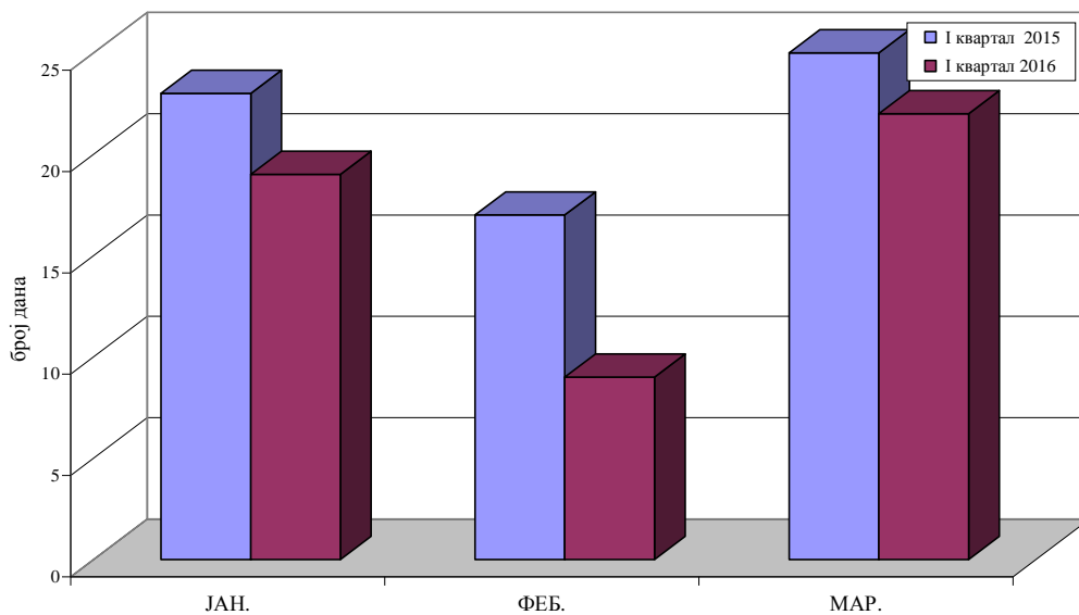
PM10 У ВАЗДУХУ АМБИЈЕНТА Мерно место: Панчево, Народна башта Упоредни приказ броја дана са концентрацијама изнад GV I квартал 2015.-I квартал 2016.
