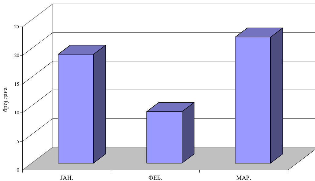
PM 10 У ВАЗДУХУ АМБИЈЕНТА Мерно место: Панчево, Народна башта Број дана са концентрацијама PM 10 изнад GV I квартал 2016.
