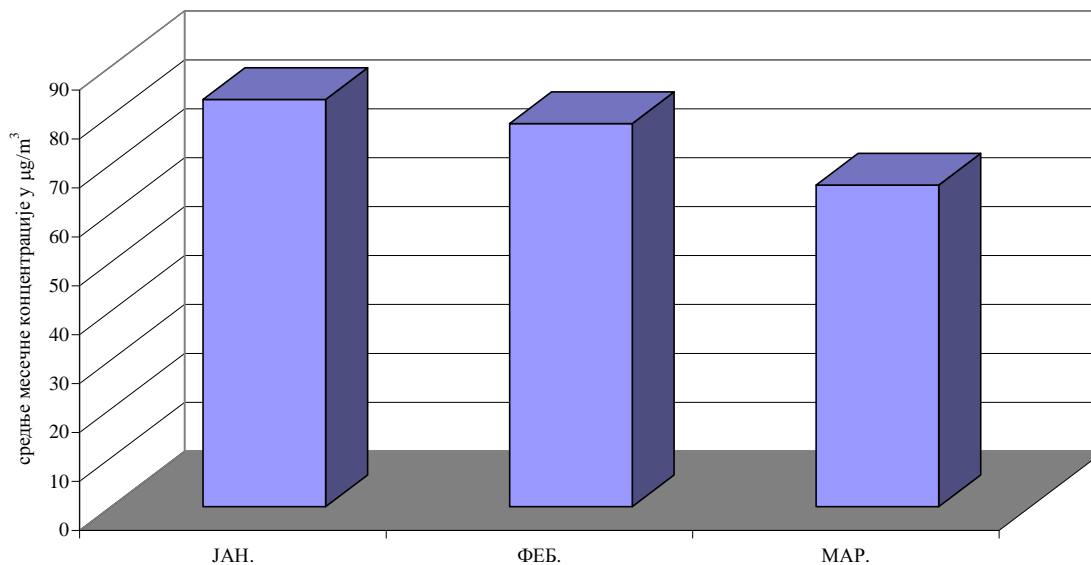
PM10 у ваздуху амбијента Мерно место: Панчево, Народна башта I квартал 2016.године Сезонска дистрибуција средњих месечних концентрација ( \mu\text{g}/\text{m}^3 ) аутоматски мониторинг
