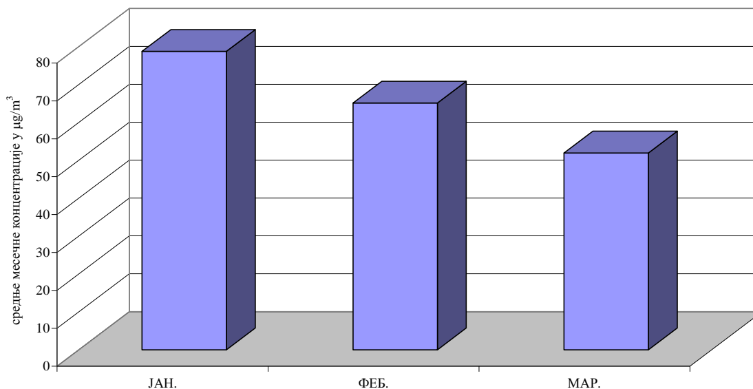
PM 2,5 у ваздуху амбијента Мерно место: Панчево, Народна башта I квартал 2016.године Сезонска дистрибуција средњих месечних концентрација ( \mu\text{g}/\text{m}^3 ) аутоматски мониторинг
