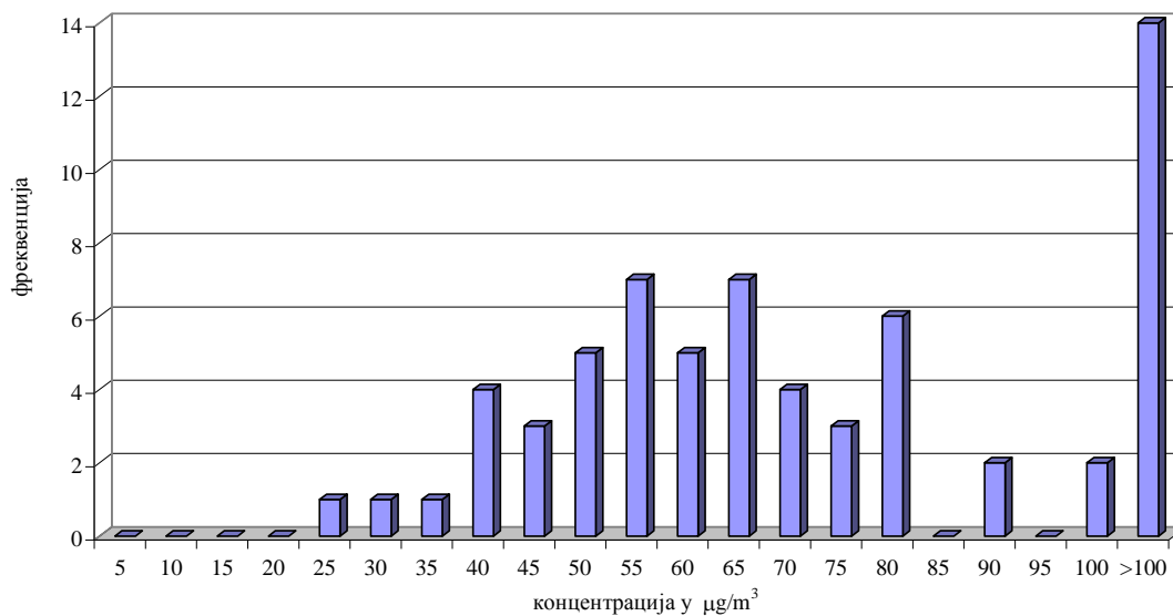
PM10 у ваздуху амбијента Мерно место: Панчево, Народна башта I квартал 2016.године Дистрибуција релативних фреквенција 24h концентрација аутоматски мониторинг
