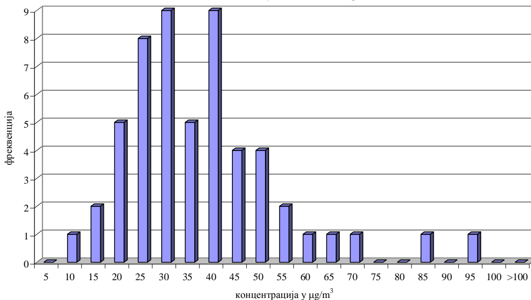
NO x у ваздуху амбијента Мерно место: Панчево, Народна башта I квартал 2016.године Дистрибуција релативних фреквенција 24h концентрација аутоматски мониторинг
