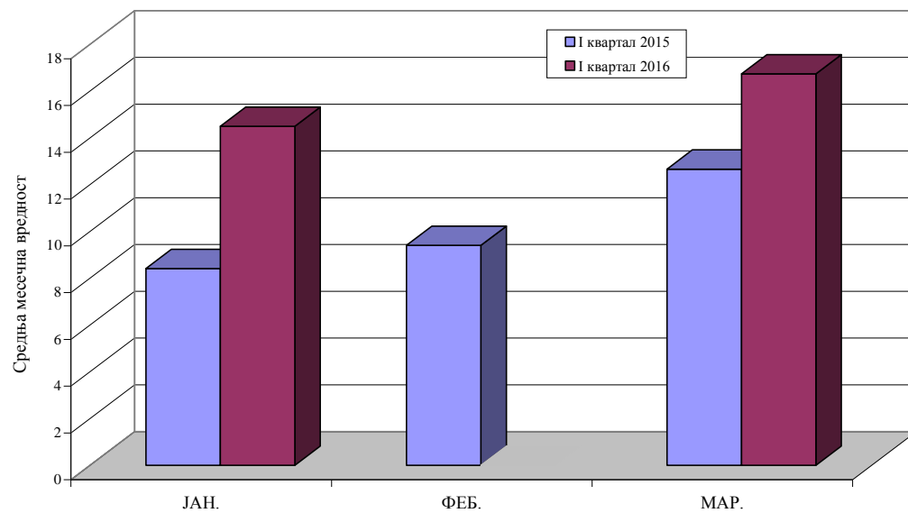
АМОНИЈАК У ВАЗДУХУ АМБИЈЕНТА Мерно место: Панчево, Народна башта Упоредни приказ просечних месечних концентрација у \mu\text{g}/\text{m}^3 I квартал 2015. - I квартал 2016.
