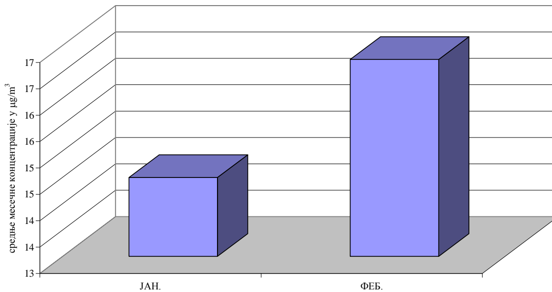
Амонијак у ваздуху амбијента Мерно место: Панчево, Народна башта I квартал 2016.године Сезонска дистрибуција средњих месечних концентрација ( \mu\text{g}/\text{m}^3 ) аутоматски мониторинг
