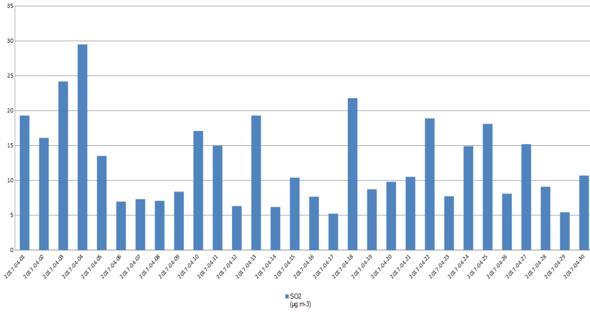
Војловица SO2
