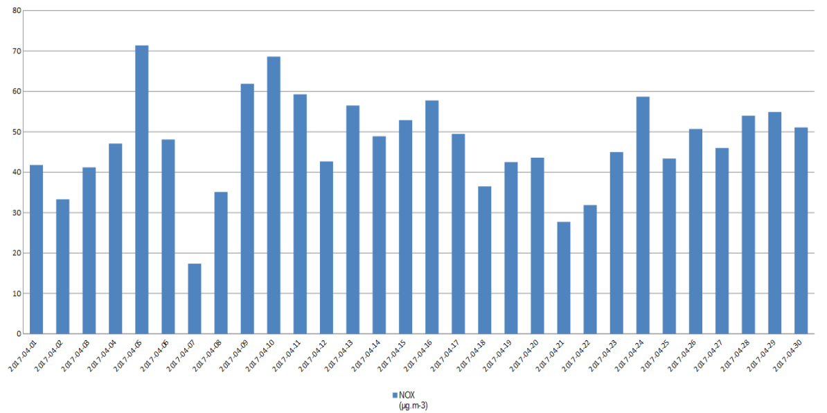
Старчево NOx
