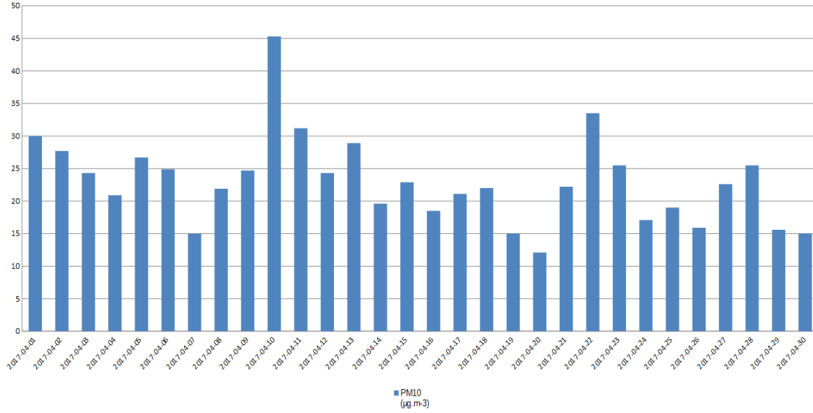
Старчево PM10
