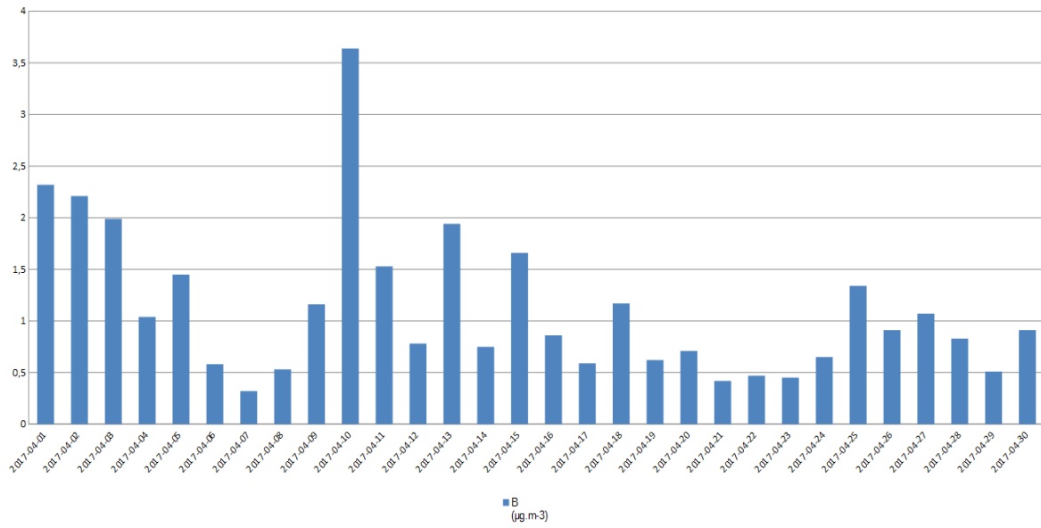
Војловица бензен
