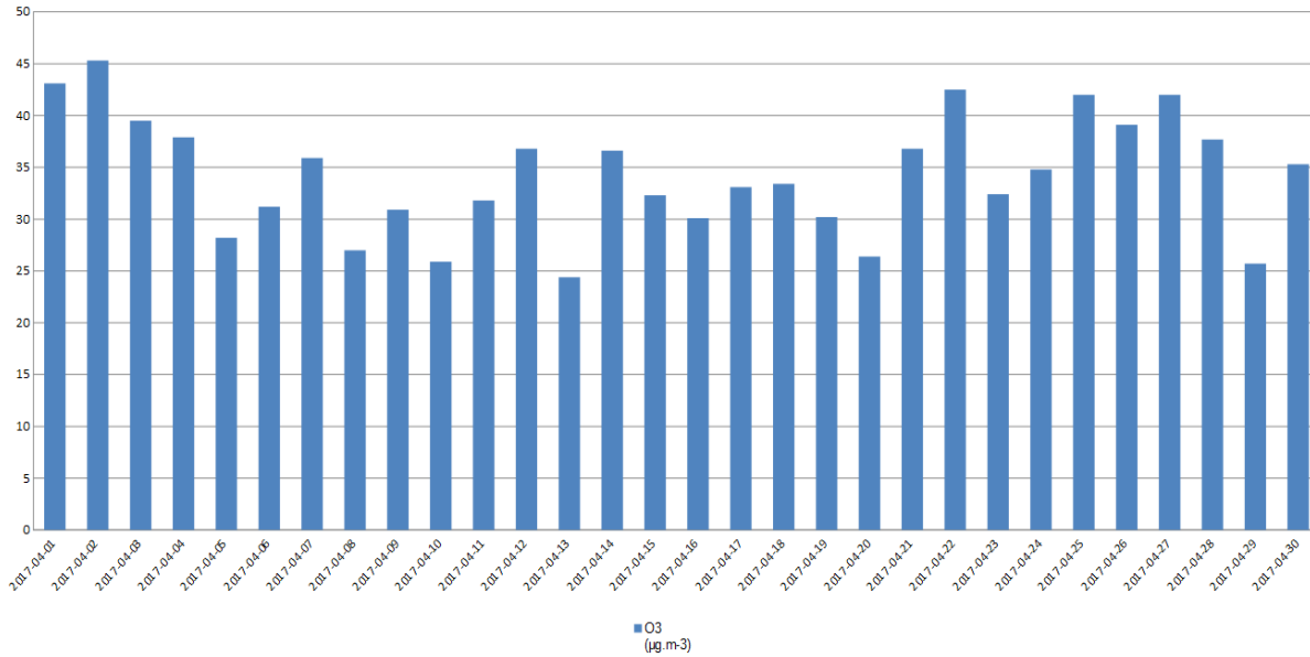
Старчево O3
