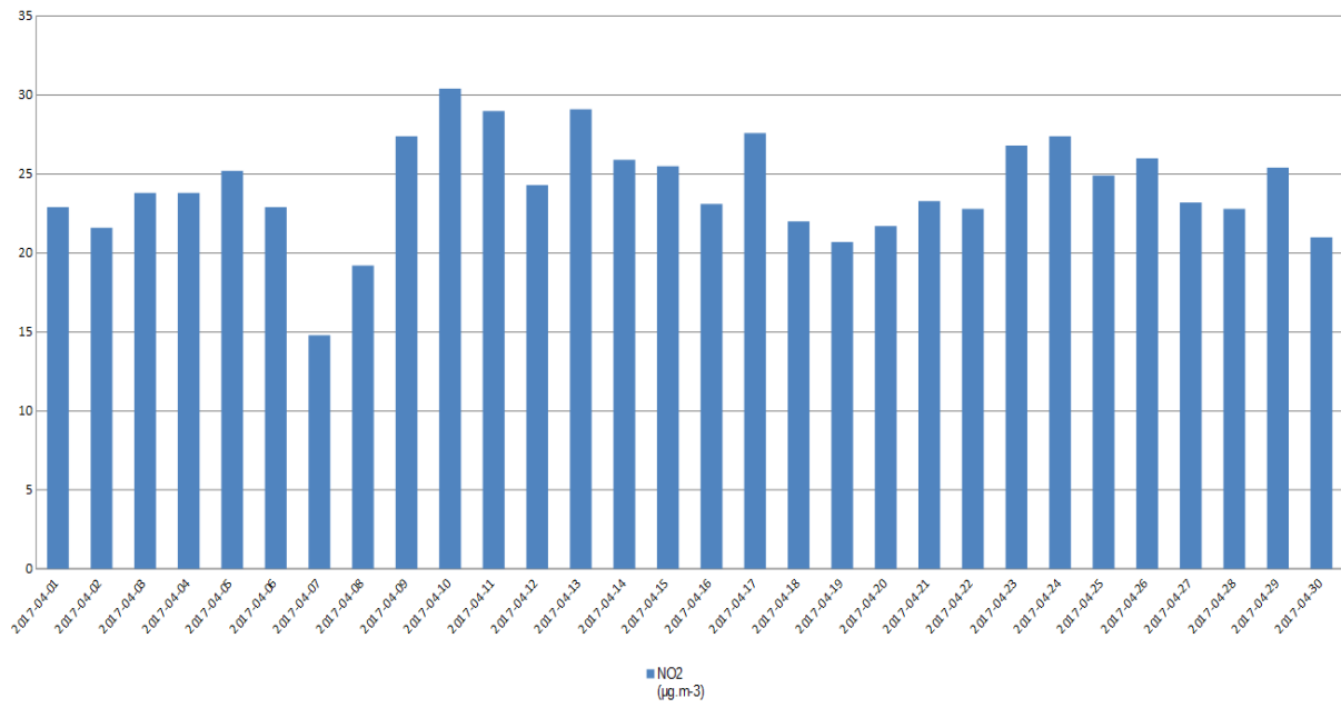
Старчево NO2
